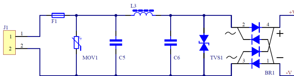
Obrázok 6.5 Vstupný filter a usmerňovací diódový mostík
