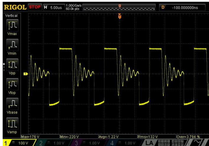
Obrázok 8.2 Priebeh napätia U_{L1} na induktore L_1
