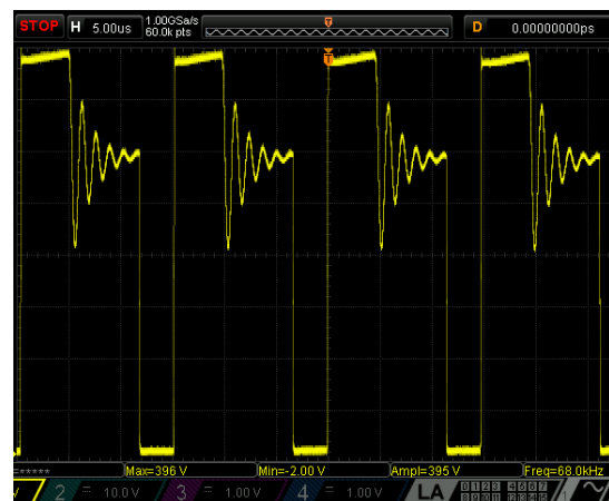
Obrázok 8.3 Napätie U_{DS} bez RC článku na D_1 (vľavo) a s RC článkom (vpravo)
