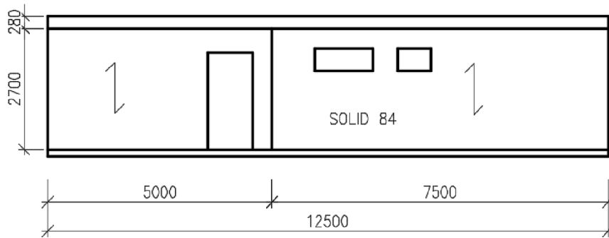
Obrázek 28 Schéma skladby panelů SOLID 84 - severní pohled
