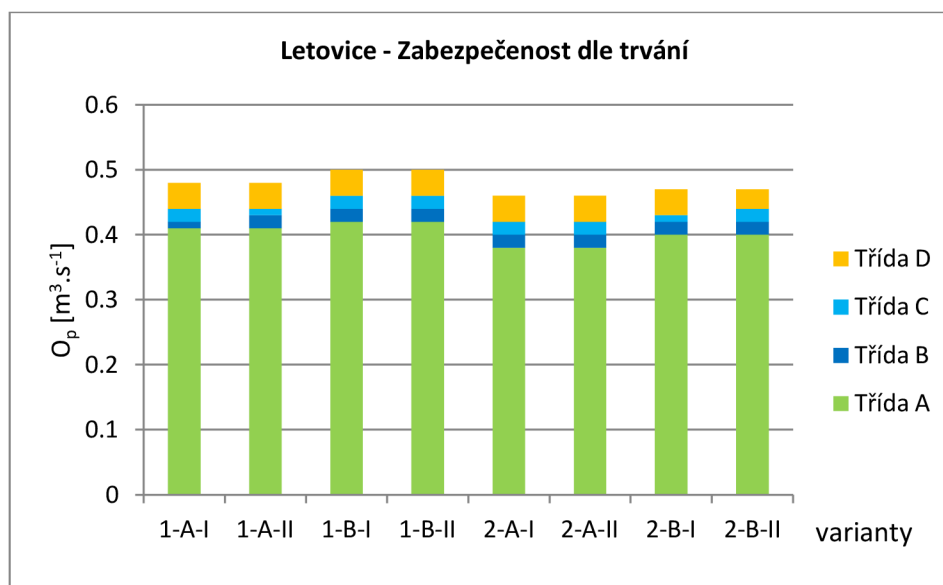
Obr. 7 Srovnání nejlepšíh odtoků z nádrže Letovice podle zabezpečení dle trvání pro 8 řešených variant
