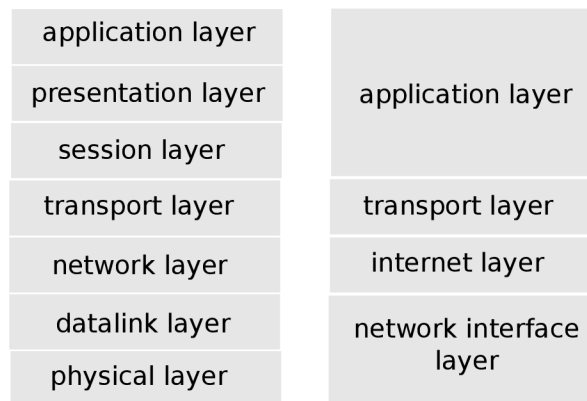
Obrázok 2.1: Model OSI a TCP/IP
