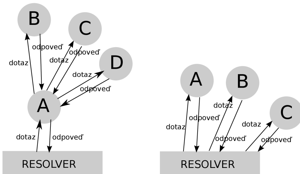
Obrázok 2.3: Príklad rekúrvizného a iteratívneho dotazovania
