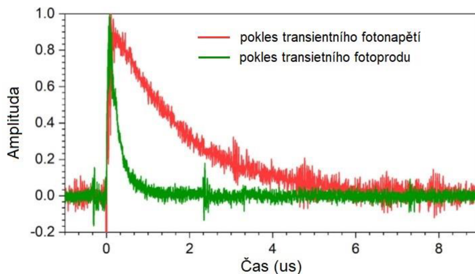
Obr. 6.4 Srovnání odchylky transientního fotoproudu a ATF při osvětlení [20]
