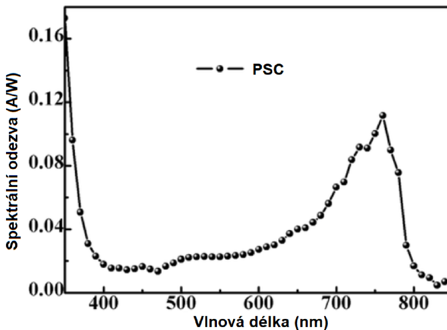
Obr. 6.15 Spektrální odezva perovskitového solárního článku \text{CH}_3\text{NH}_3\text{PBI}_3 [17]
