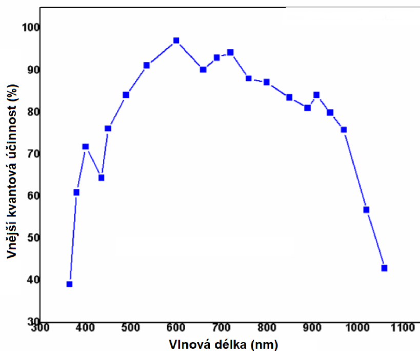
Obr. 6.14 Vnější kvantová účinnost EQE křemíkového solárního článku [16]
