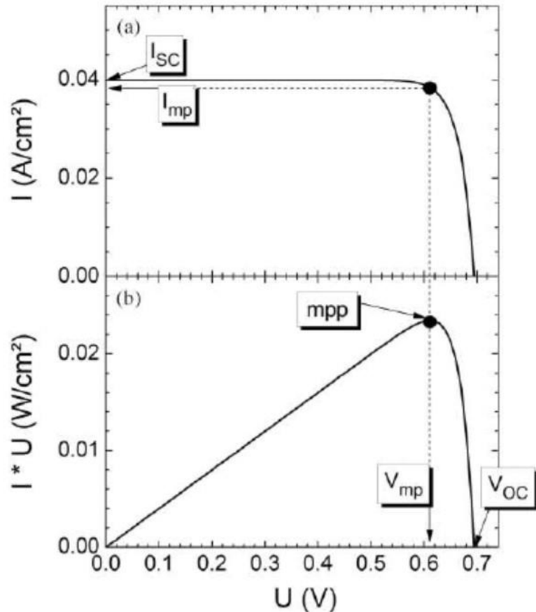
Obr. 6.12 Příklad zatěžovací charakteristiky [5]
