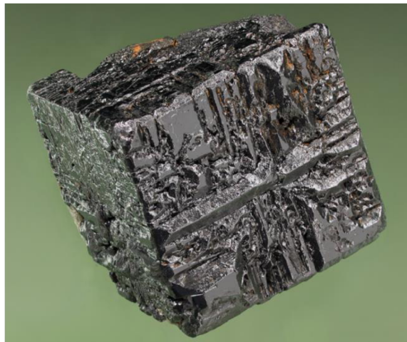
Obr. 2.1 Minerál perovskitu [2]
