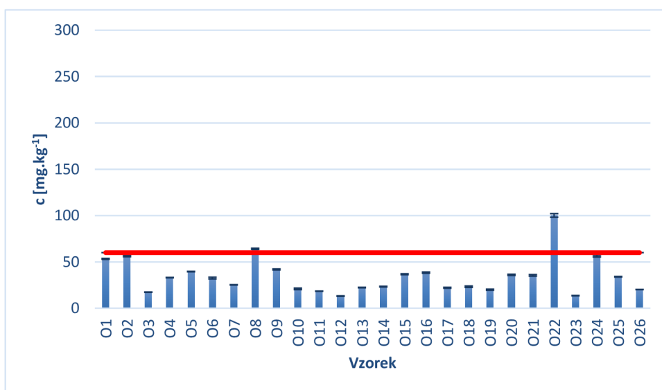
Graf č. 23: Hodnoty koncentrací olova pro jednotlivá odběrová místa z Ostravy
