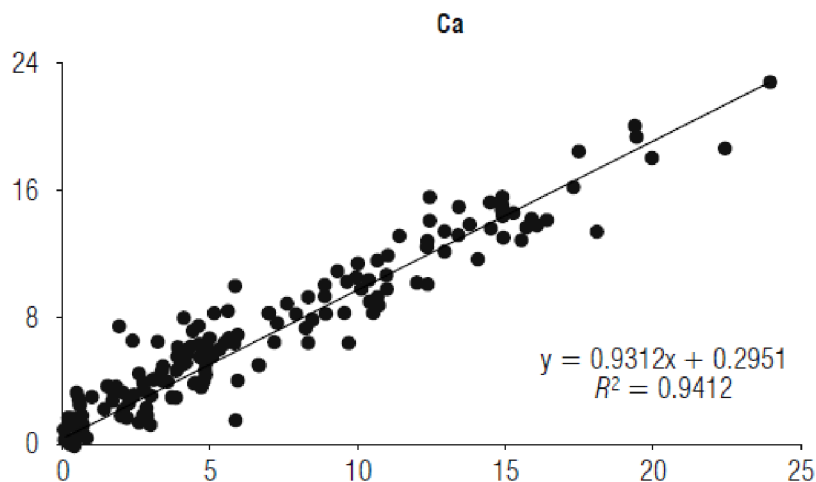
Graf č. 4: Korelace predikčních a změřených hodnot vlastností půdy pro vápník [49]
