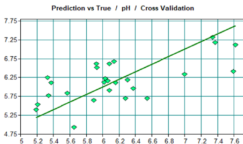
Graf č. 27: Korelační model pH se vzorky z lokality Ostrava
