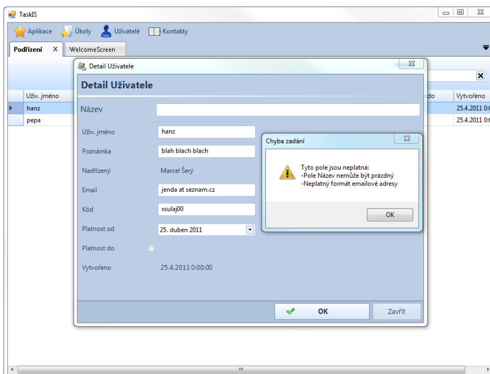
Obrázek 10: Funkce validátorů
