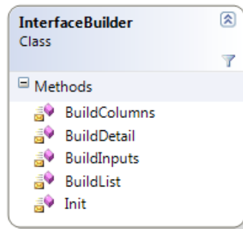
Obrázek 3: Třída InterfaceBuilder
