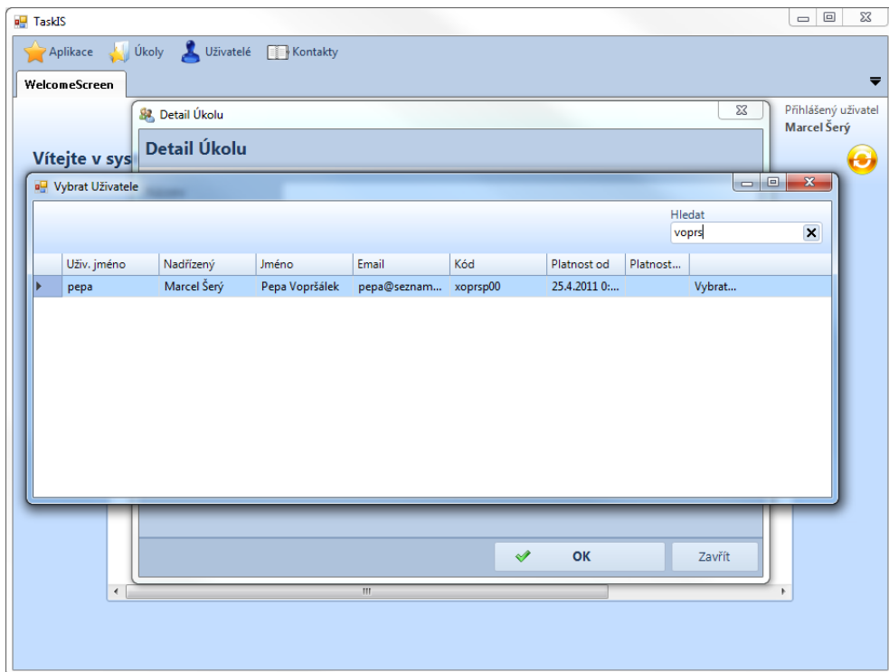
Obrázek 6: Výběr uživatele
