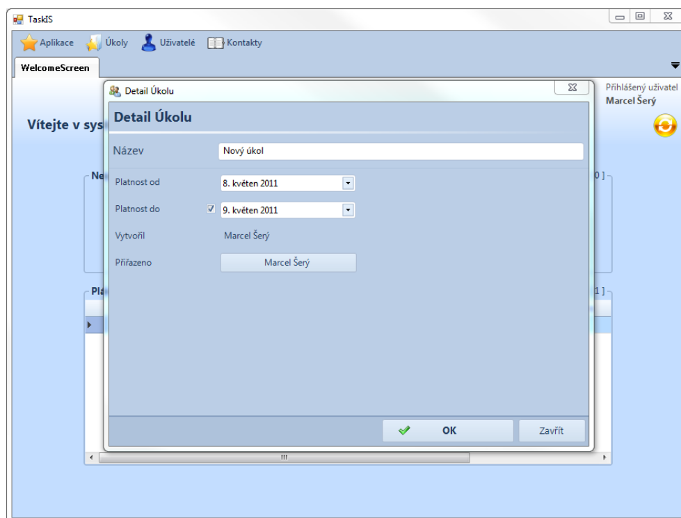
Obrázek 5: Nový úkol
