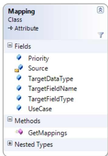
Obrázek 2: Třída Mapping
