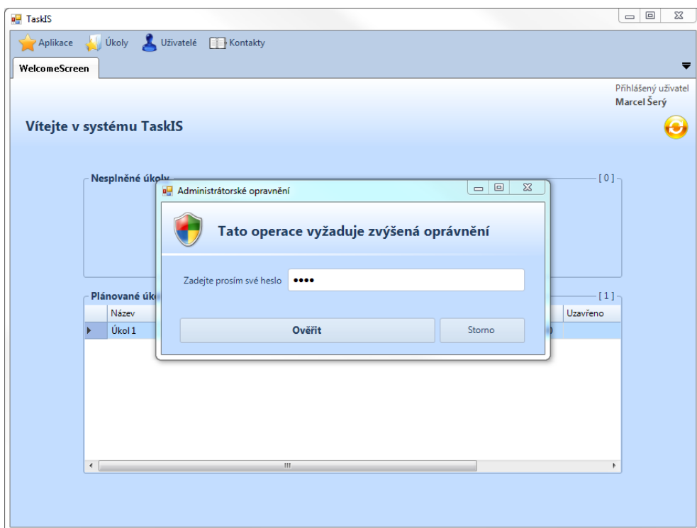
Obrázek 7: Zvýšená oprávnění
