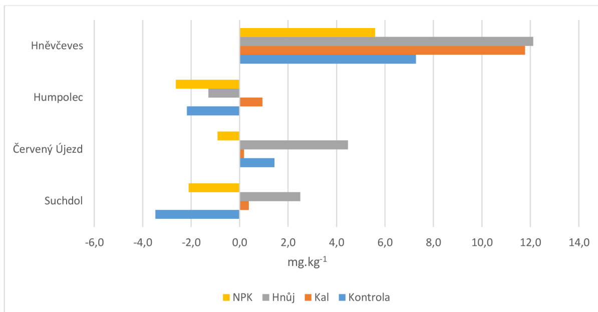
Graf č. 3: Bilance obsahu hořčíku v půdě ve vodném výluhu od roku 1996 do roku 2017 (mg.kg -1 )
