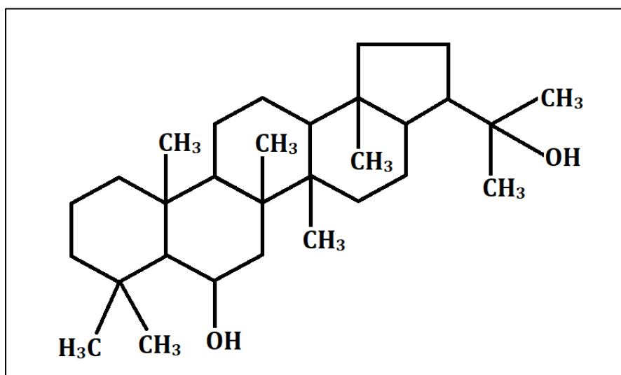
Obr. 8: Vzorec zeorinu.
