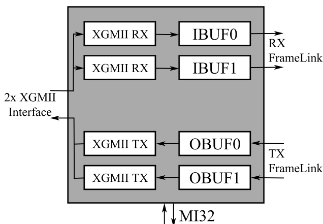
Obrázek 4.4: Znázornění struktury síťového modulu (pro 10 Gbps síťová rozhraní)
