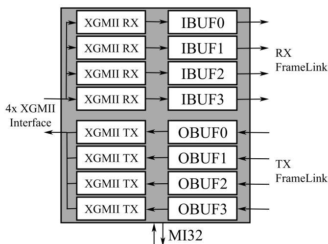
Obrázek 5.2: Znáznornění struktury síťového modulu pro kartu NetFPGA-10G
