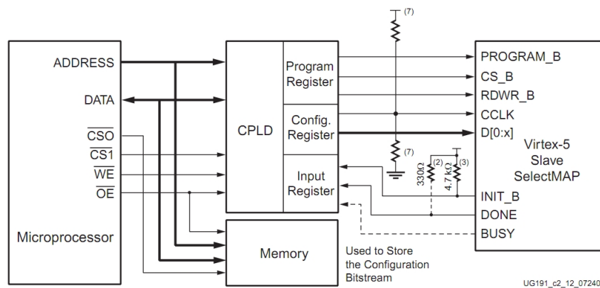
Obrázek 2.7: Schéma zapojení Slave SelectMAP [32]
