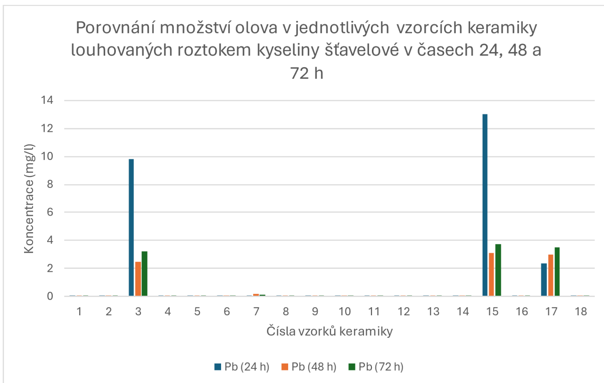
Graf 12 Porovnání množství olova v jednotlivých vzorcích keramiky louhovaných roztokem kyseliny šťavelové v časech 24, 48 a 72 h. Zajímavostí je, že se nám koncentrace olova ve výluzech u vzorku 3 a 15 mezi 24 a 48 hodinami snižovala.
