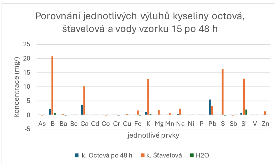
Graf 20 Porovnání jednotlivých prvků ve výluhu kyselinou octovou, šťavelovou a vody ve vzorku 15 po 48 h
