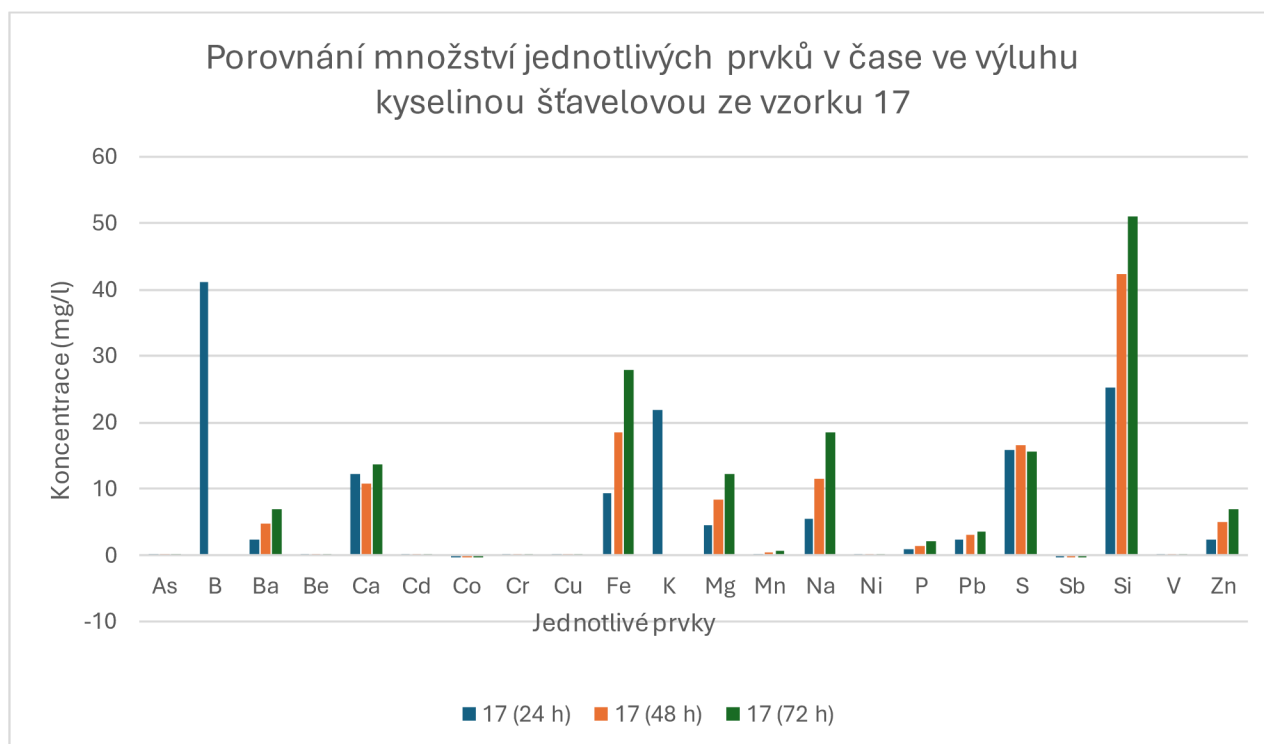
Graf 11 Porovnání množství jednotlivých prvků v čase ve výluhu kyselinou šťavelovou ze vzorku 17. Oprotu glazurám 3 a 15 se nám ve vzorku 17 nejvíce uvolňoval křemík.
