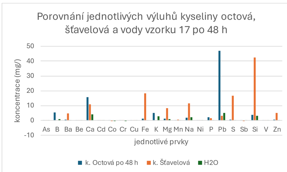
Graf 19 Porovnání jednotlivých prvků ve výluhu kyselinou octovou, šťavelovou a vody ve vzorku 17 po 48 h
