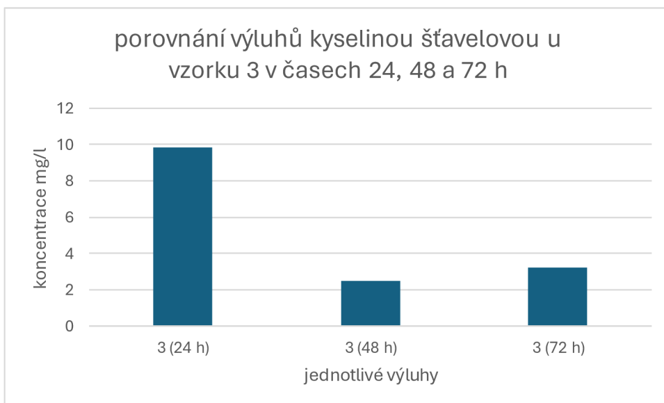
Graf 13 Porovnání množství olova ve výluzech kyselinou šťavelovou u vzorku 3 v časech 24, 48 a 72 hodin.
