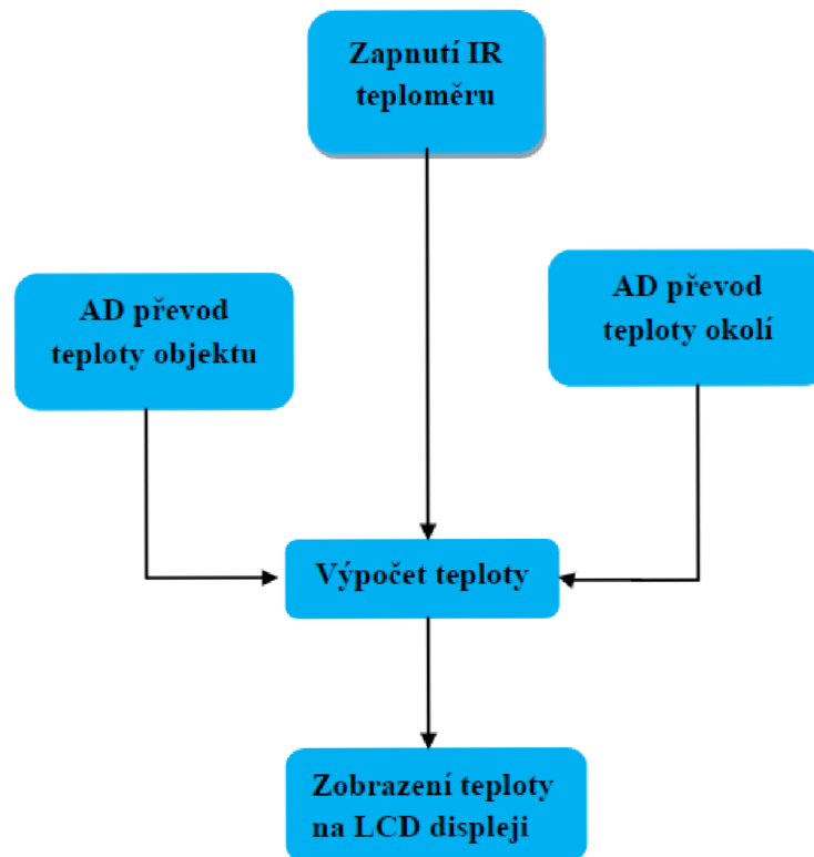
Obrázek 26 : Schéma programového řešení
