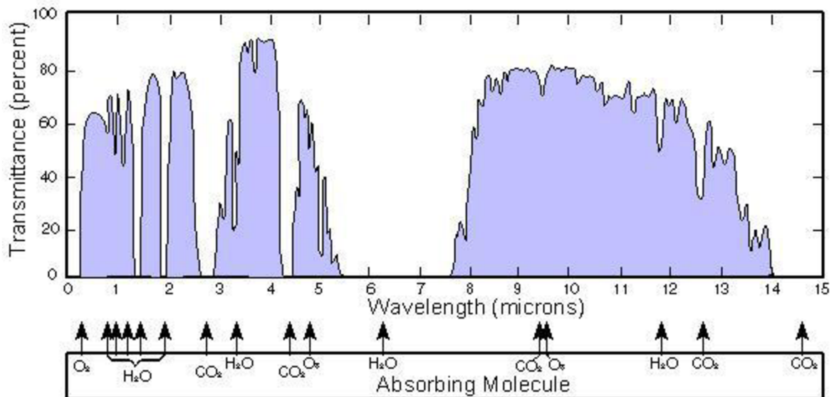
Obrázek 10 : Závislost atmosférické propustnosti na vlnové délce [29]
