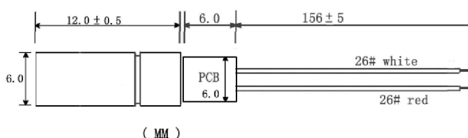
Obrázek 20 : Laserový modul LM650-D6, [11]
