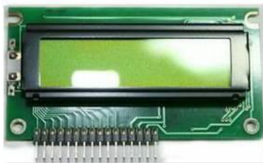
Obrázek 21 : Displej PC1602-LRU-FWA-B-Q, [10]
