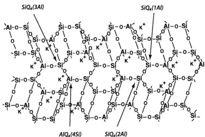
Obrázek 5: Teoretický model plně zesíťovaného geopolymery (K-poly(sialate-silixo)) podle prof. Davidovitse
