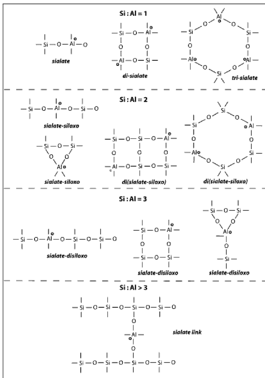
Obrázek 6: Nákrisy slouženin podle Davidovitse [20]
