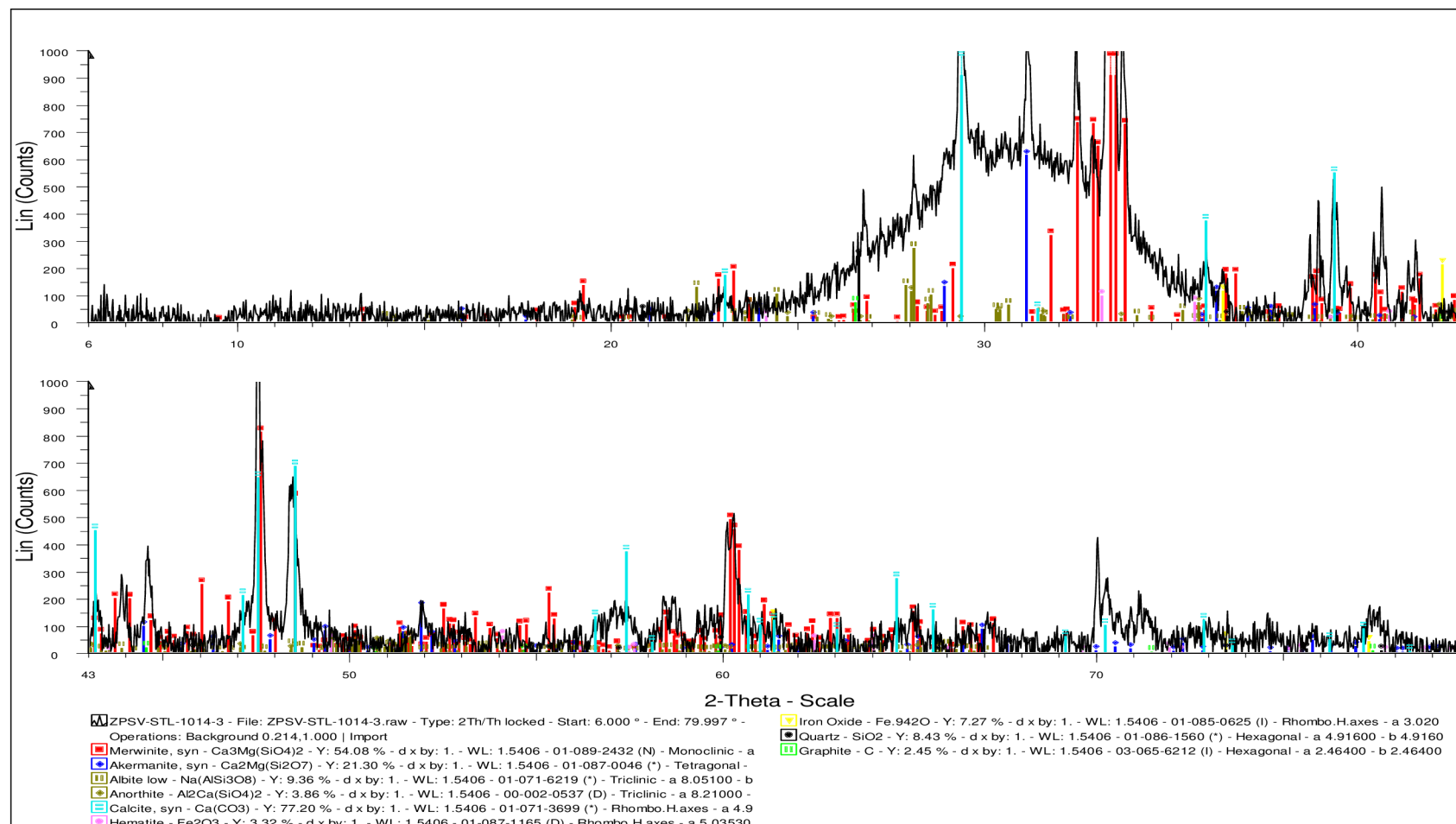
Obrázek 5: rentgenový difraktogram Ocelářské strusky Třinec 1.7.2008
