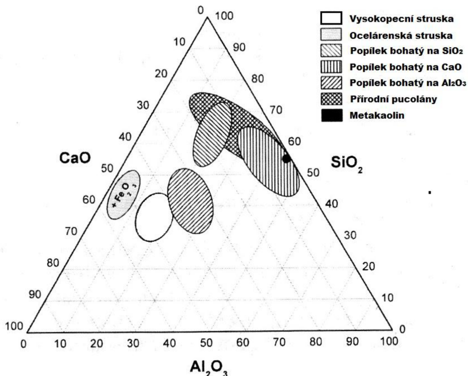
Obrázek 11: Diagram zobrazující přibližné zastoupení oxidů důležitých materiálů pro výrobu geopolymerů [1]
