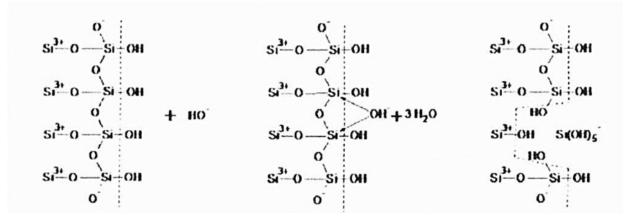
Obrázek 9: Schéma alkalického rozpouštění křemíku [1]
