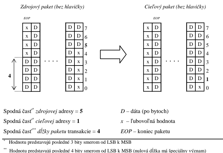
Obrázok 6.6: Princíp prerovňovania dát v generátore paketov internej zbernice.
