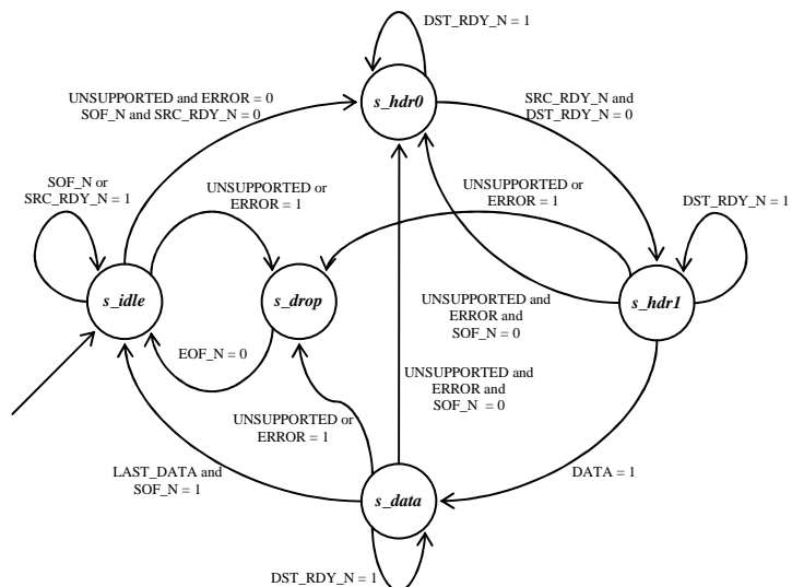
Obrázok 6.4: Riadiaci automat dekodéra paketov systémovej zbernice.
