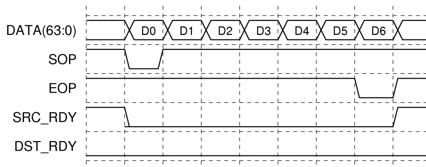
Obrázok 5.3: Priebeh transakcie na internej zbernici.
