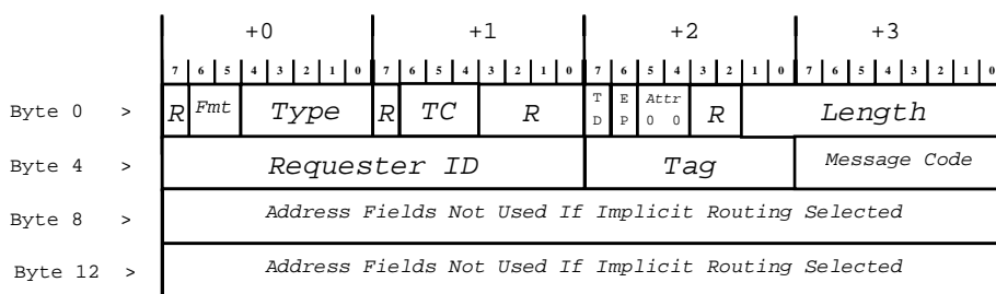
Obrázok 3.10: Formát hlavičky transakcie typu Message.
