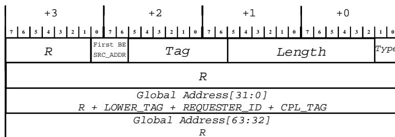
Obrázok 6.8: Formát hlavičky obecného paketu v TX smere.
