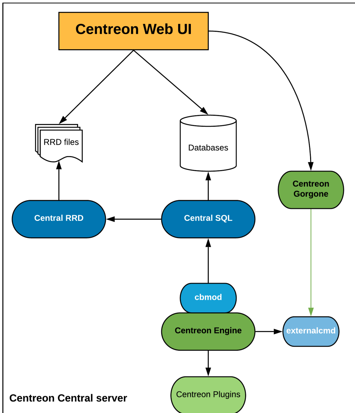
Obrázek č. 19: Diagram jednoduché architektury (35)
