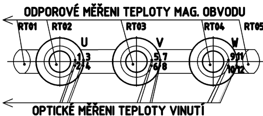
Obr. 5-9 Schéma instalace nitronádobového měření teplot blokových transformátorů [5]
