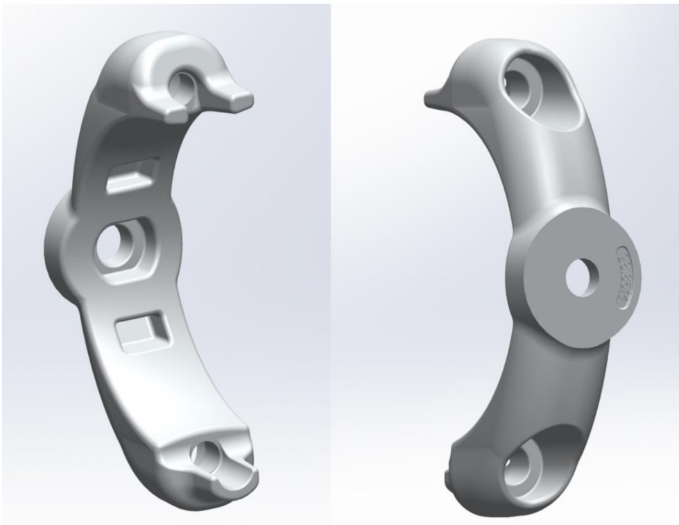
Obr. 2: 3D model odlitku ze dvou pohledů
