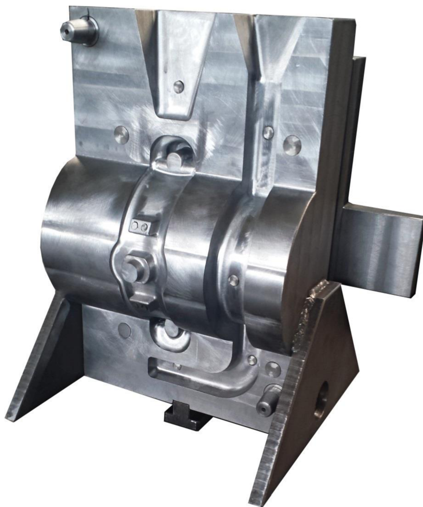
Obr. č. 16: Pohled na vyrobenou pohyblivou polovinu formy
