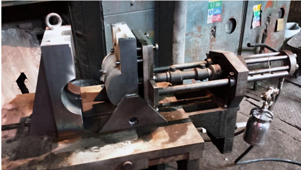
Obr. č. 18: Upevněná a otevřená forma na kokilovém licím stroji KS-2
