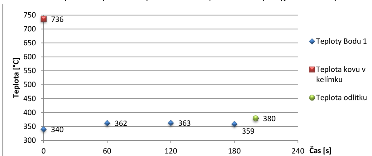
Obr. č. 23: Průběh teploty v bodě 1
