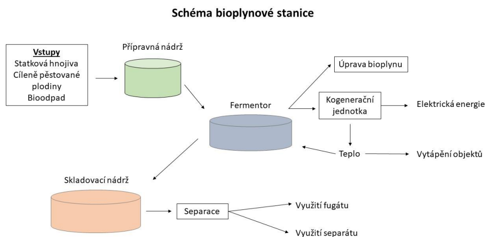
Obr. 1 Schéma bioplynové stanice (Autor V. Wanča)
