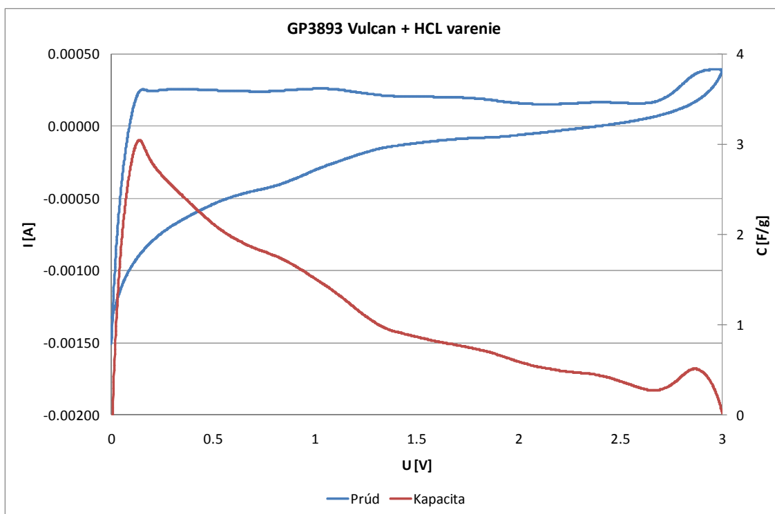
Obr.11 Cyklická voltmetria GP3893 Vulcan+HCL s ďalším varením
