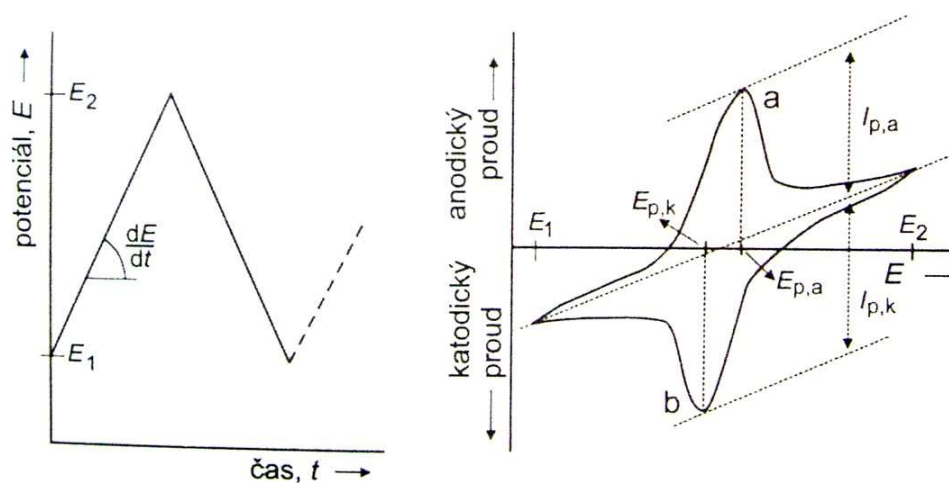
Obr.5: Potenciálový program a prúdová odozva pri cyklickej voltametrii. V príklade je na cyklickom voltamograme vidieť, ako sú produkty vzniknuté oxidáciou (špička a) a pri opačnom smere potenciálové zmeny redukované (špička b).
