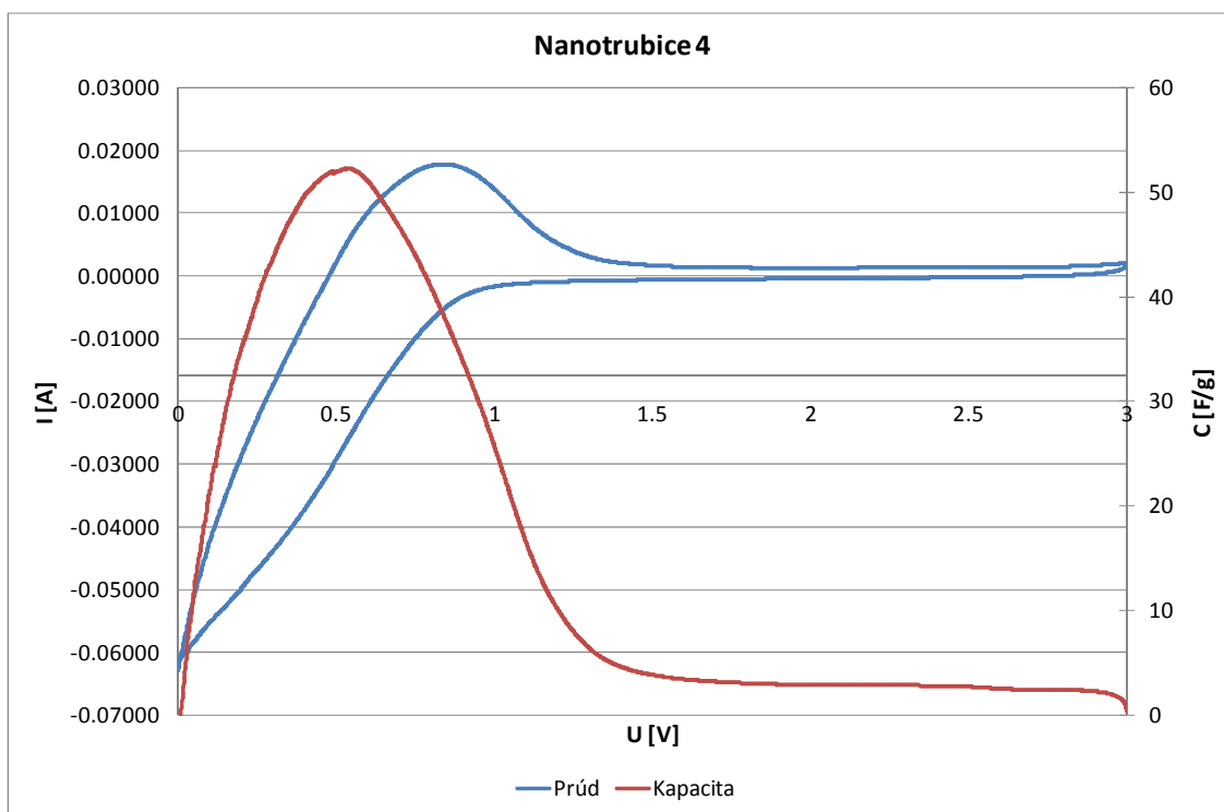
Obr.22 Cyklická voltametria Nanotrubice 4
