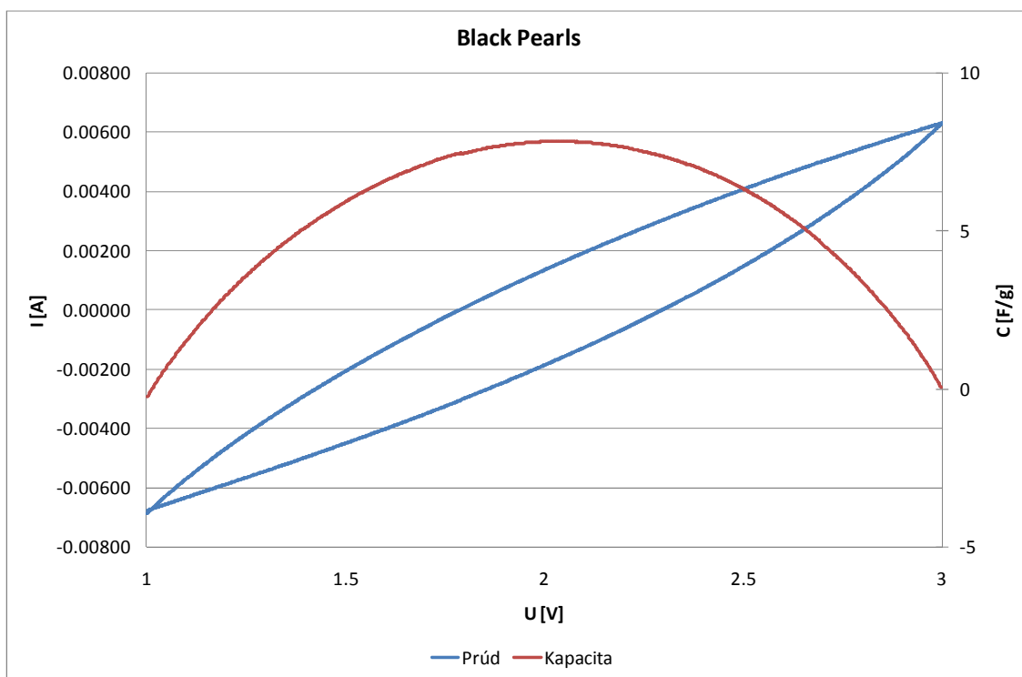
Obr.14 Cyklická voltametria Cabot Black Pearls 2000
