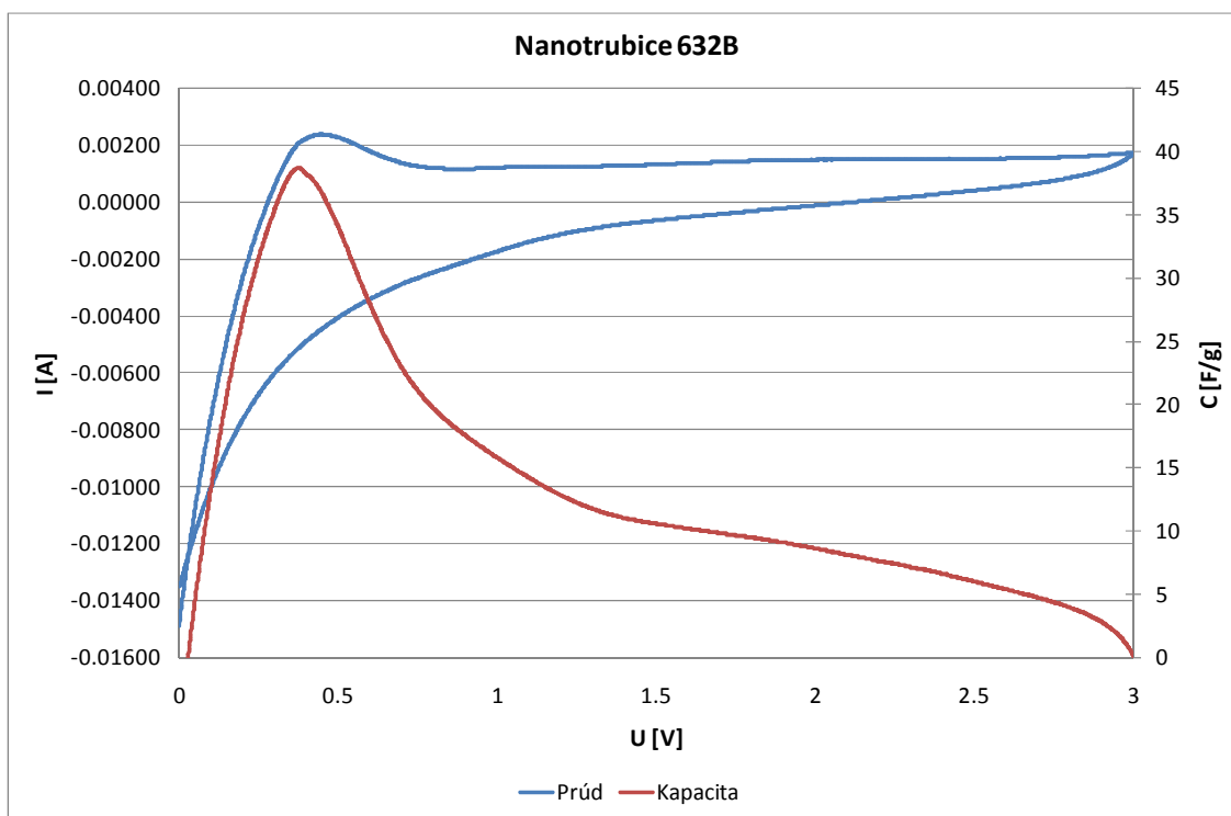
Obr.16 Cyklická voltmetria Nanotrubička 632B
