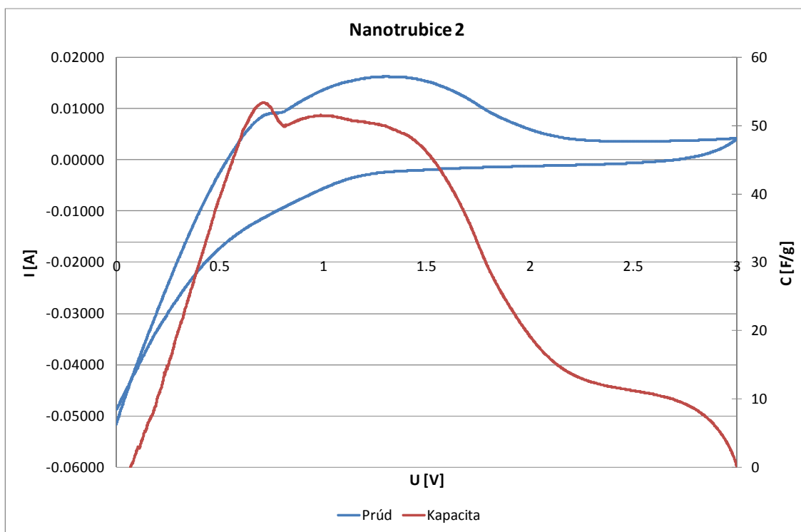
Obr.20 Cyklická voltametria Nanotrubice 2
