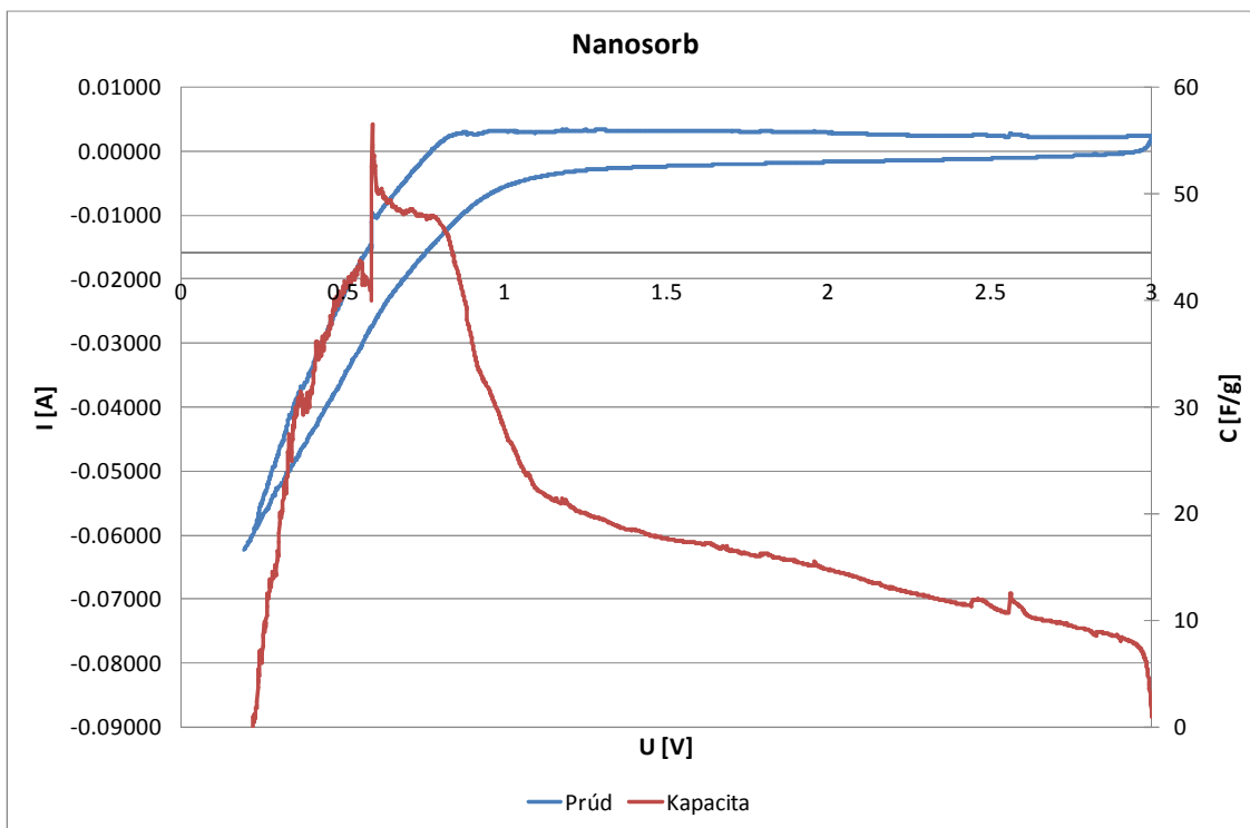
Obr.18 Cyklická voltametria Nanosorbu
