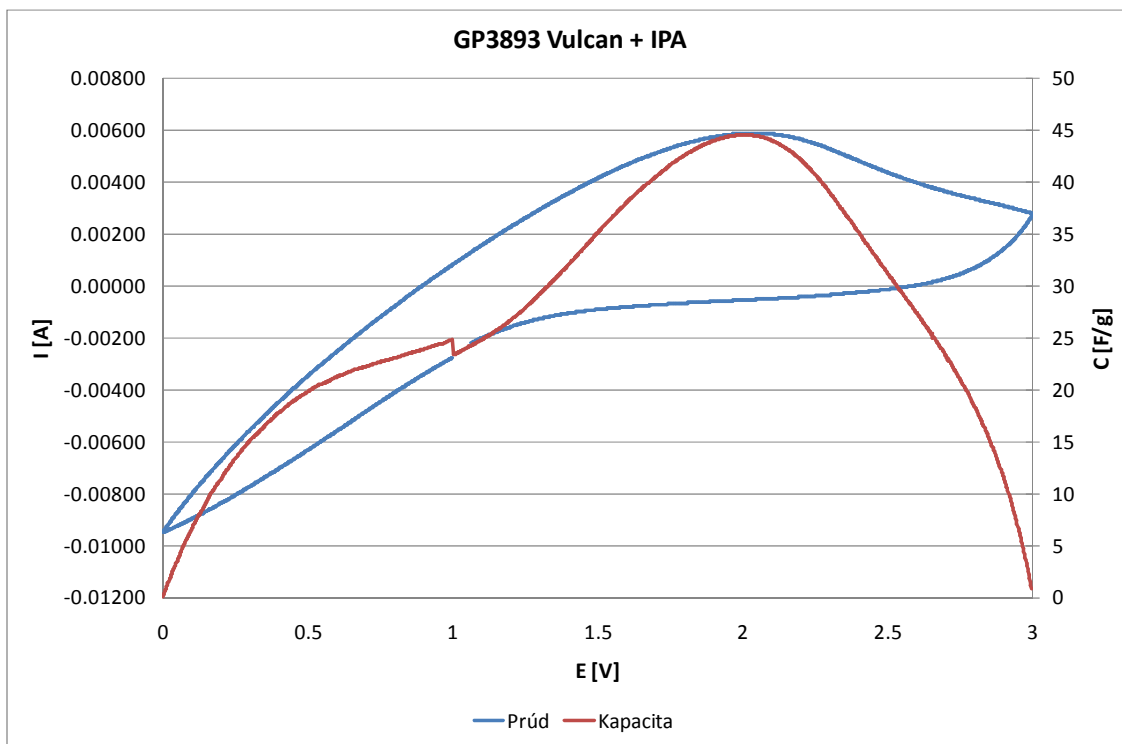
Obr.8 Cyklická voltametria GP3893 Vulcan s použitím izopropylalkoholu
