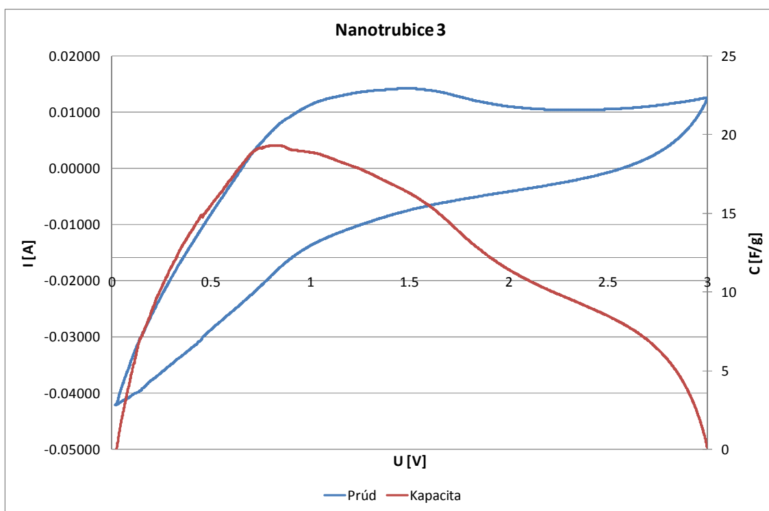
Obr.21 Cyklická voltametria Nanotrubice 3
