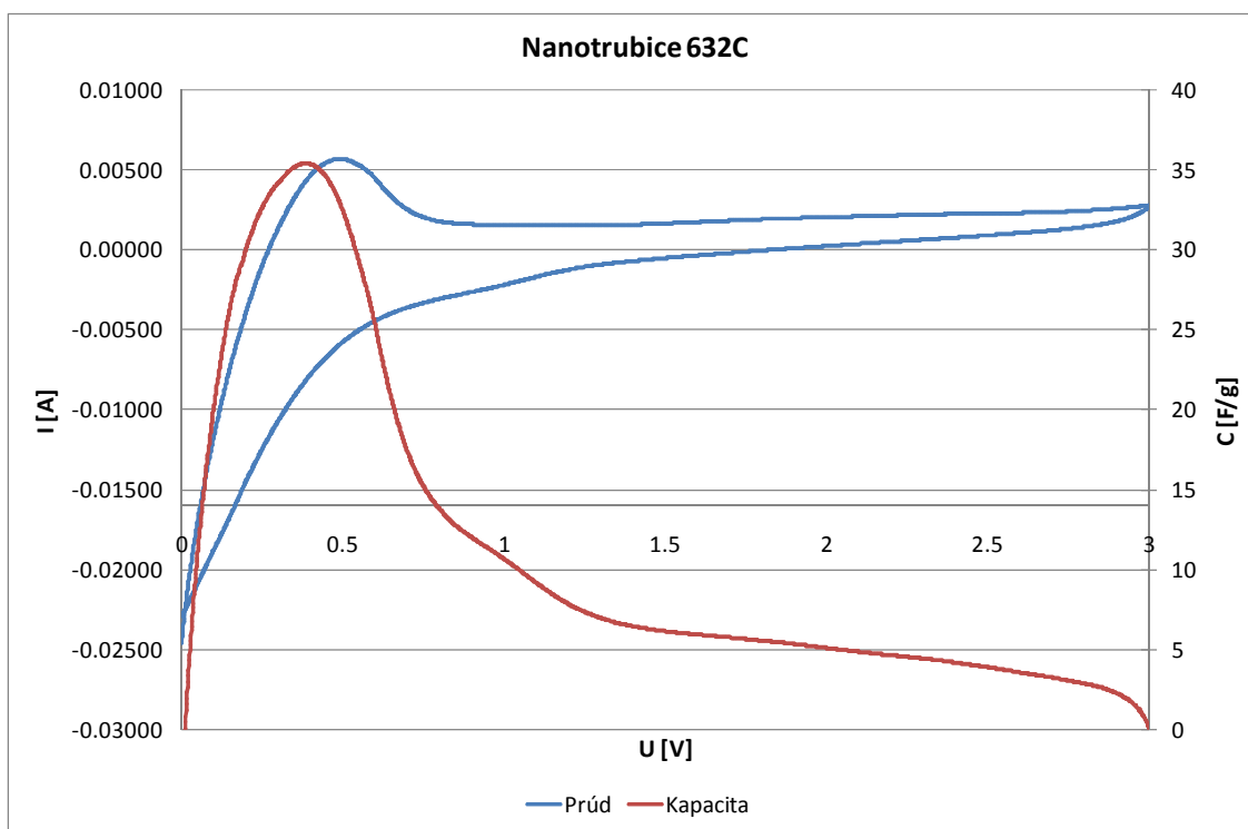
Obr.17 Cyklická voltmetria Nanotrubička 632C
