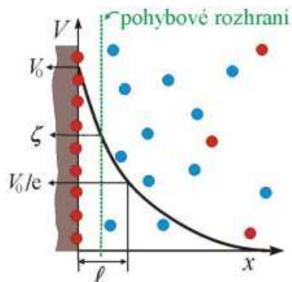
Obr.2 Gouy – Chapmanov model elektrickej dvojvrstvy
