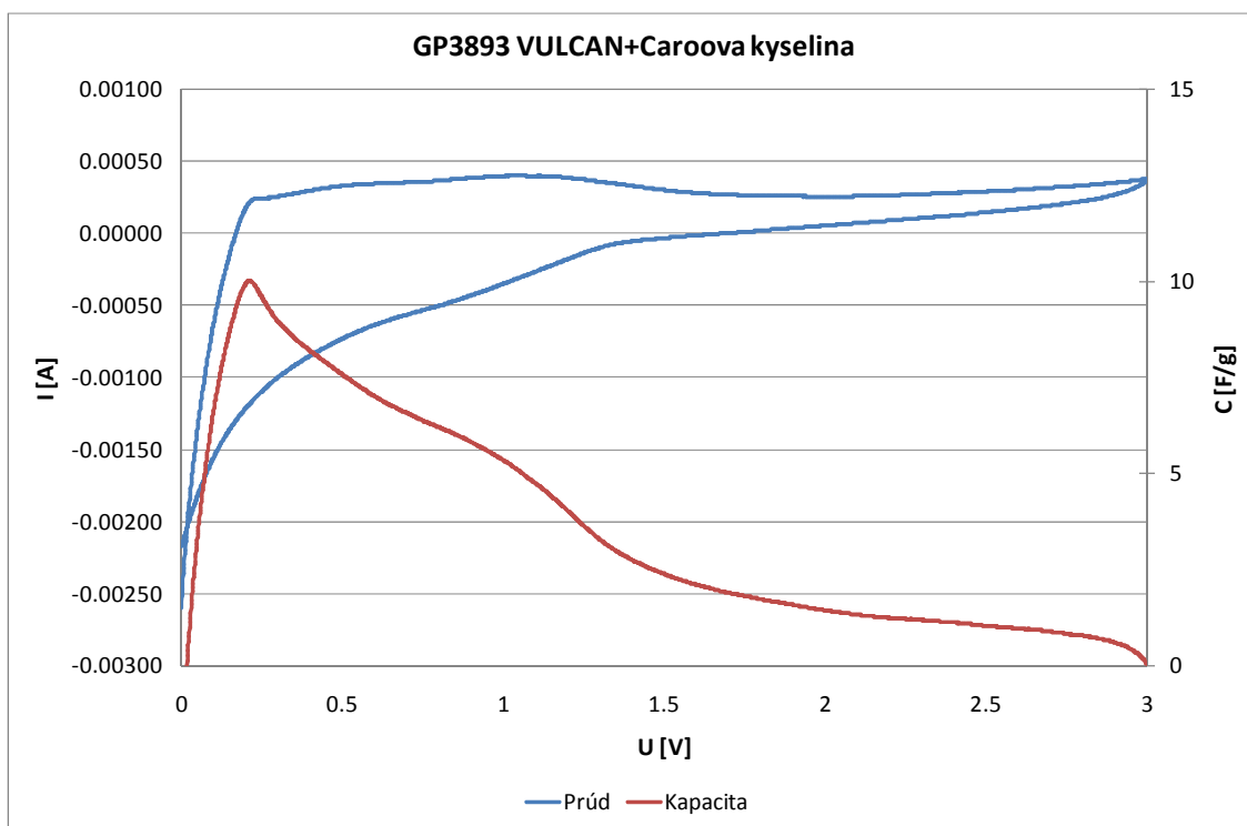
Obr.12 Cyklická voltmetria GP3893 Vulcan+Caroova kyselina
