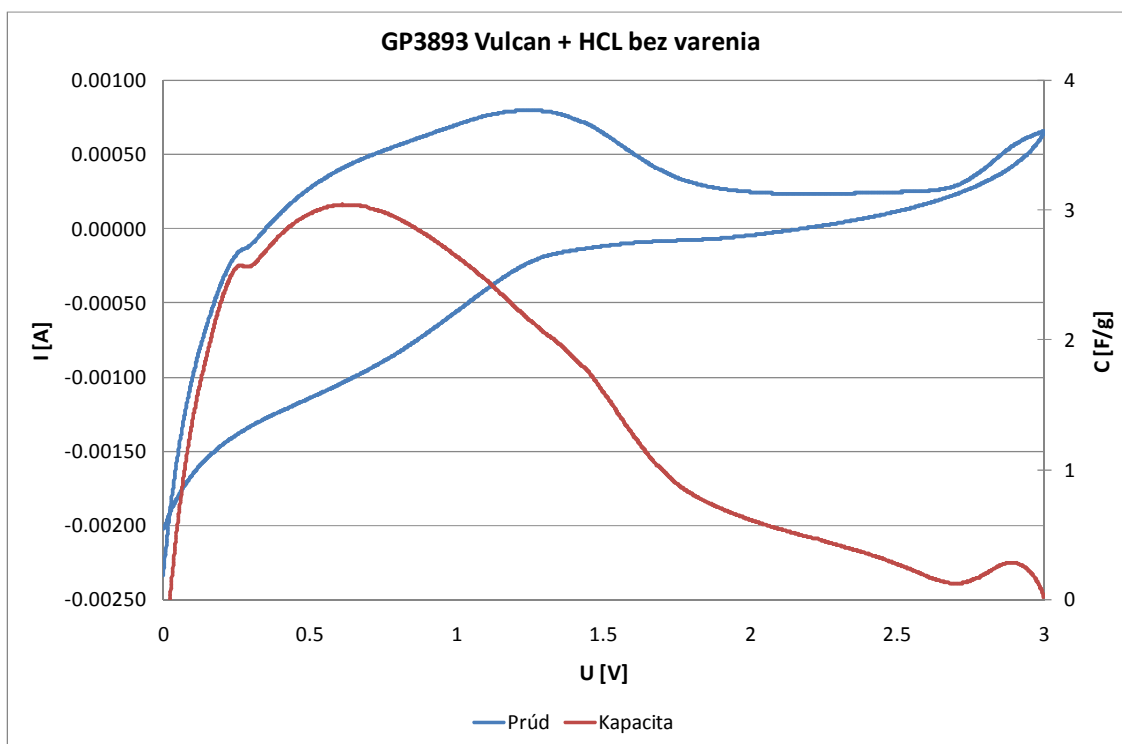
Obr.10 Cyklická voltmetria GP3893 Vulcan+HCL bez ďalšieho varenia
