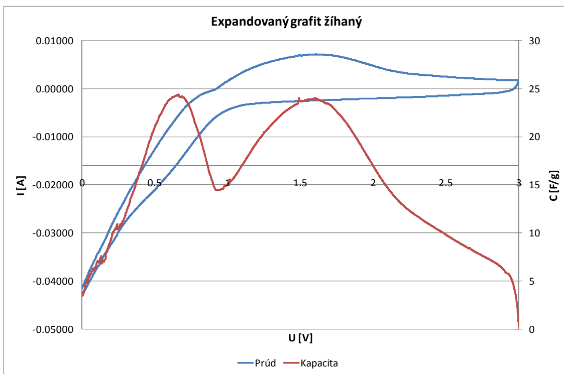
Obr.15 Cyklická voltametria Expandovaného žíhaného grafitu
