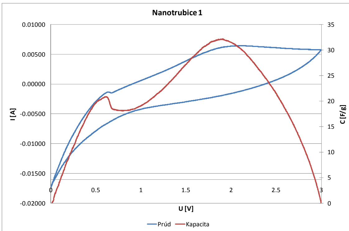
Obr.19 Cyklická voltametria Nanotrubice 1
