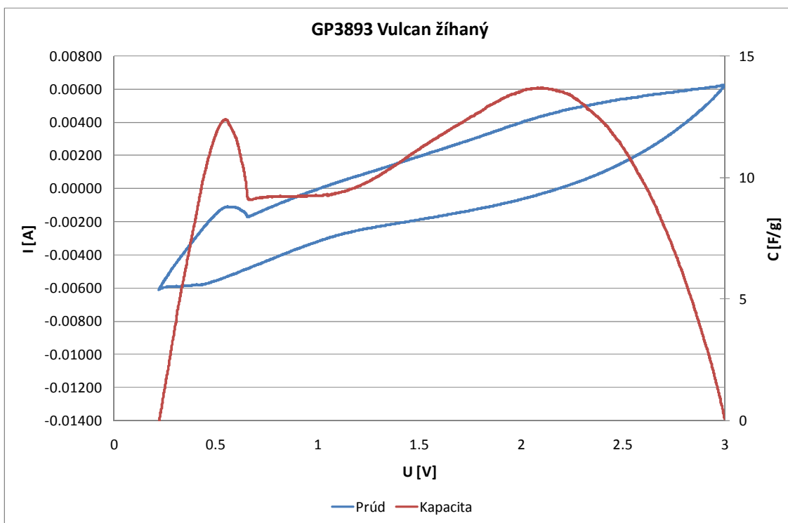
Obr.9 Cyklická voltametria GP3893 Vulcan žíhaný
