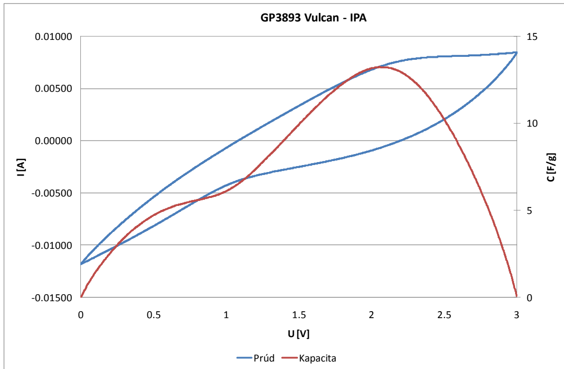
Obr.7 Cyklická voltametria GP3893 Vulcan bez použitia izopropylalkoholu
