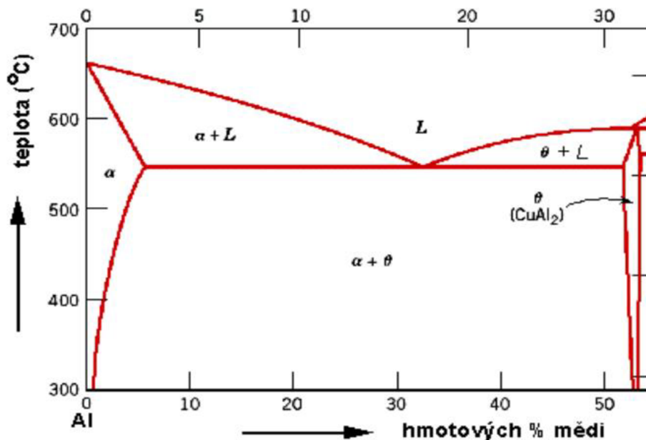
Obrázek 3: Diagram binární soustavy Al-Cu s výraznou změnou rozpustnosti [12]
