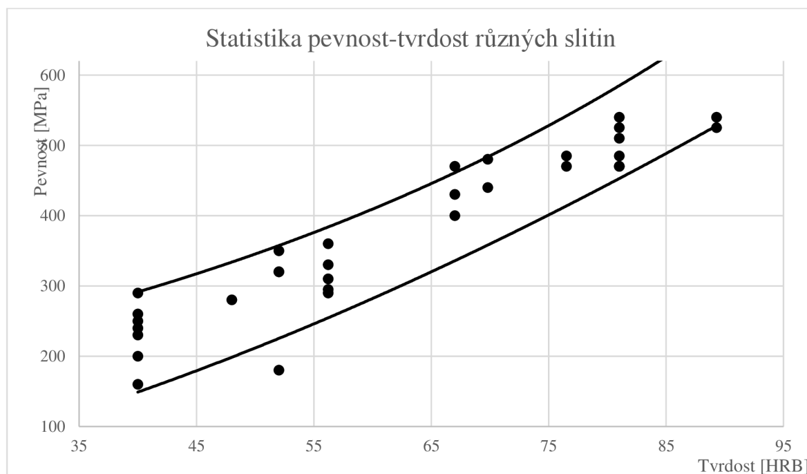
Graf 15: Pás hodnot tvrdost-pevnost pro různé slitiny
