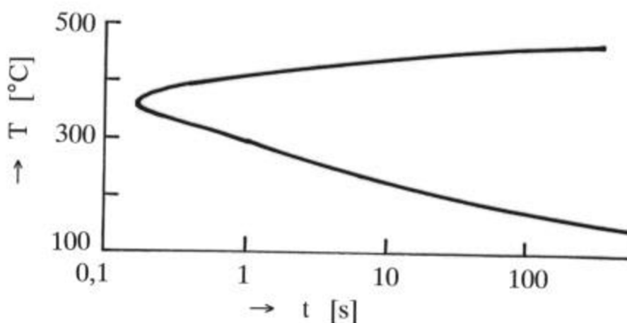
Obrázek 5: C křivka slitiny 2024 [12]
