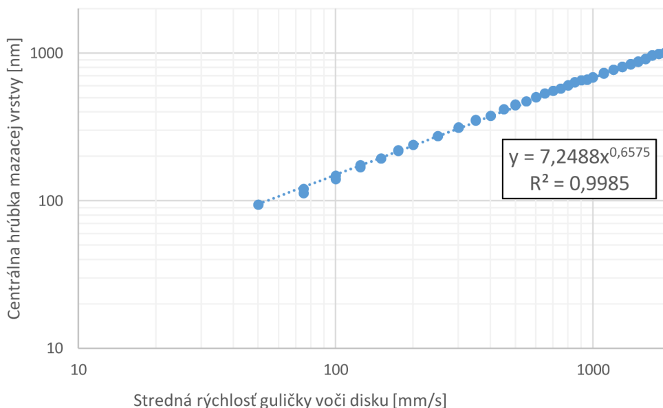
Obr. 25 Graf závislosti centrálnej hrúbky maziva na strednej rýchlosti guľičky
