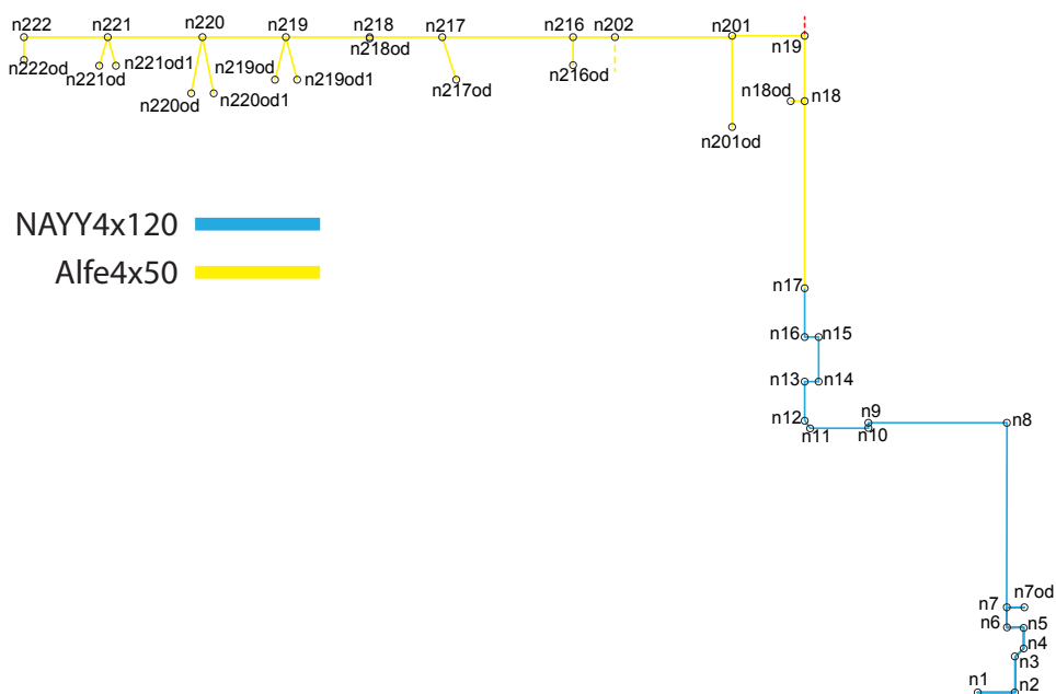
Obr. 7.9: Přenosová trasa mezi uzly n_1 a n_{222}
