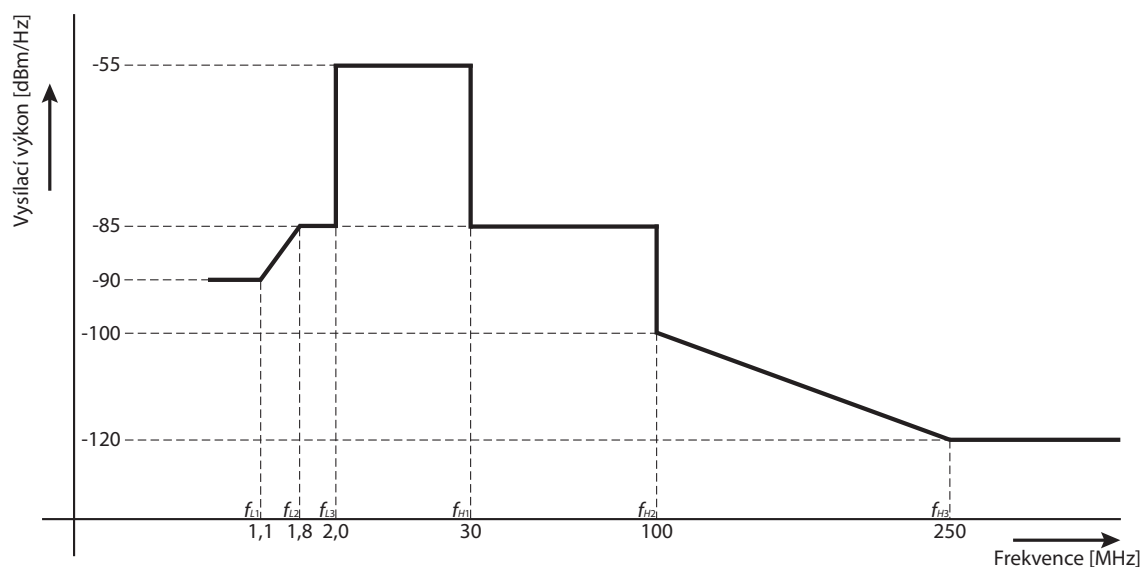
Obr. 4.1: Regulace vysílacího výkonu podle specifikace G.9964
