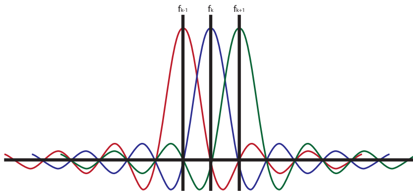
Obr. 3.1: Spektrum OFDM
