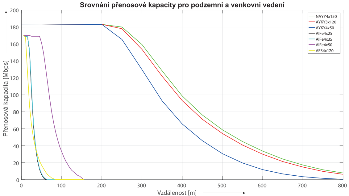
Obr. 5.3: Srovnání přenosové kapacity pro podzemní a venkovní vedení
