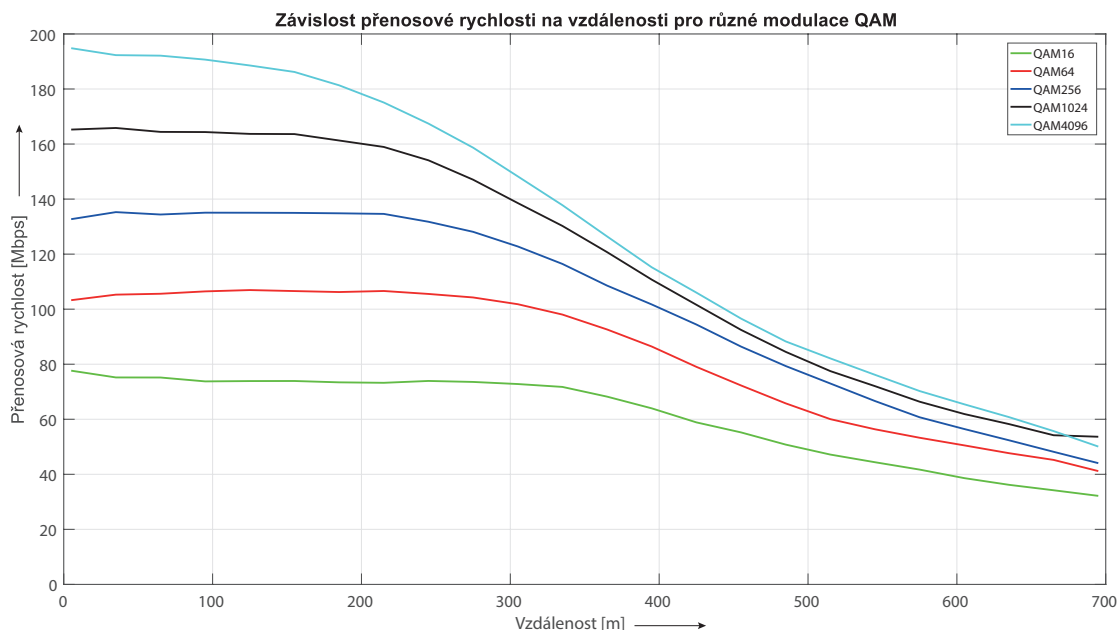
Obr. 4.6: Závislost přenosové rychlosti na vzdálenosti pro různé modulační schémata QAM
