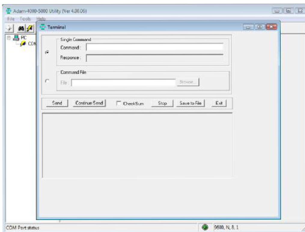
Obr. 6.11: Okno terminálu
