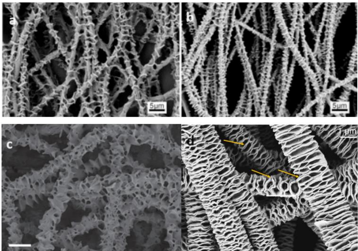
Obr. č. 9: Příklady snímků z rastrovacího elektronového mikroskopu různých vláken s postprocesní úpravou typu shish-kebab: (a) PCL/pentylacetát (Jing et al. 2014); (b) PCL/kyselina octová (Jing et al. 2014); (c) PCL/kyselina octová/voda (Wang et al. 2017); (d) PLA/xylen (Xie et al. 2020). Měřítka představují u snímků (a-c) 5 mikrometrů a u snímku (d) 1 mikrometr.
