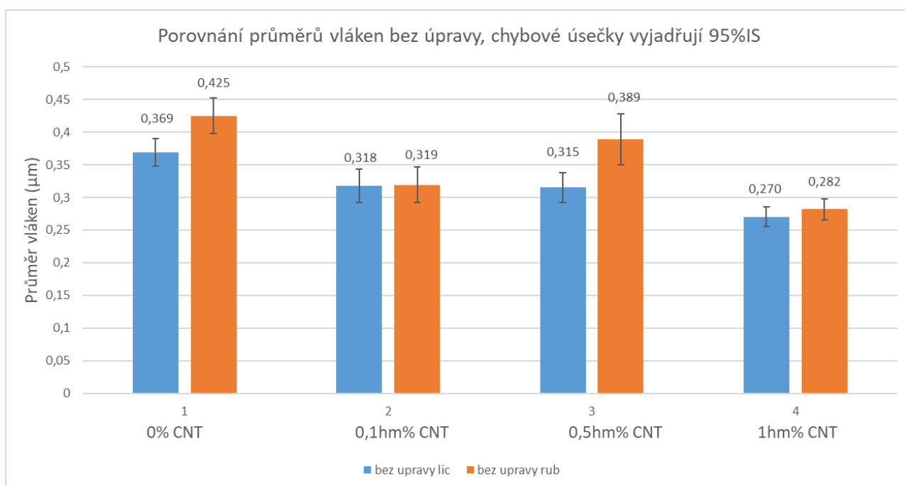
Graf č.1: Porovnání průměrů nanovláken bez postprocesní úpravy zředěným polymerním roztokem
