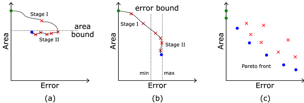
Obrázek 2.20: Aproximační strategie: (a) zdrojově orientovaná, (b) chybově orientovaná (c) víceúčelová. Obrázek přejet z [18]
