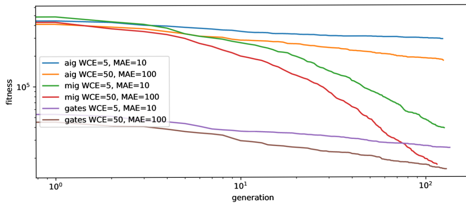
Obrázek 6.12: hodnota funkce fitness v průběhu generací
