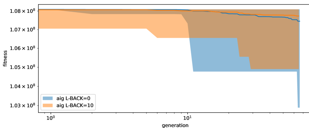
Obrázek 6.20: hodnota funkce fitness v průběhu generací (l-back=0 -> unlimited)
