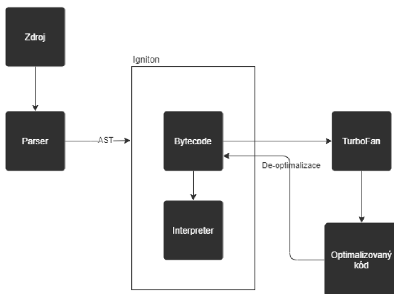
Obrázek 11 Proces kompilace ve V8 engine. Adaptováno
