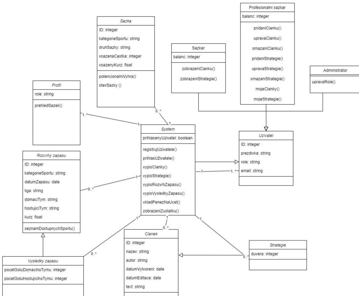
Obrázek 28 Diagram tříd
