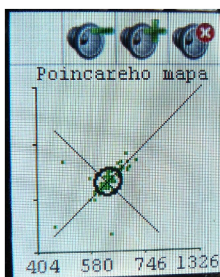
Obr. 2.7: Vykreslená Poincarého mapa
