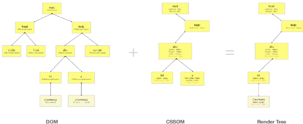
Obrázek 8 – Render Tree (13)
