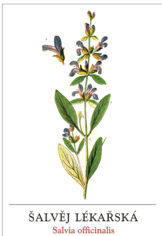
Obrázek č. 8: šalvěj lékařská (1 – část rostliny, 2 – list, 3 – květ) [34]
