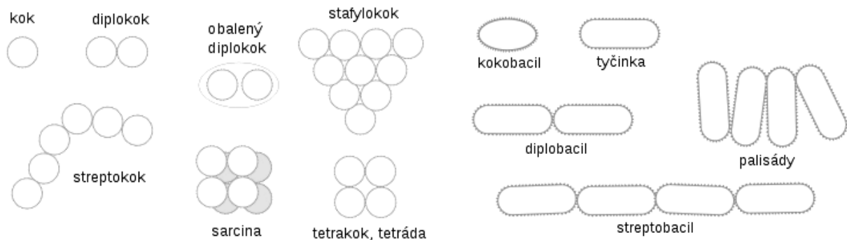
Obrázek č. 7: Tvary bakterií [36]
