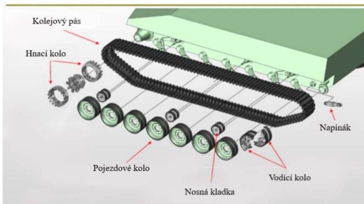
Obr. 9 Schéma pásového pohybového ústrojí [50]
