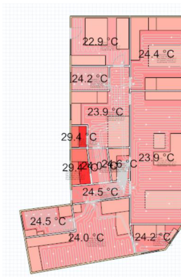
obr. 27 Vytápěcí systém s analýzou teploty podlahy
