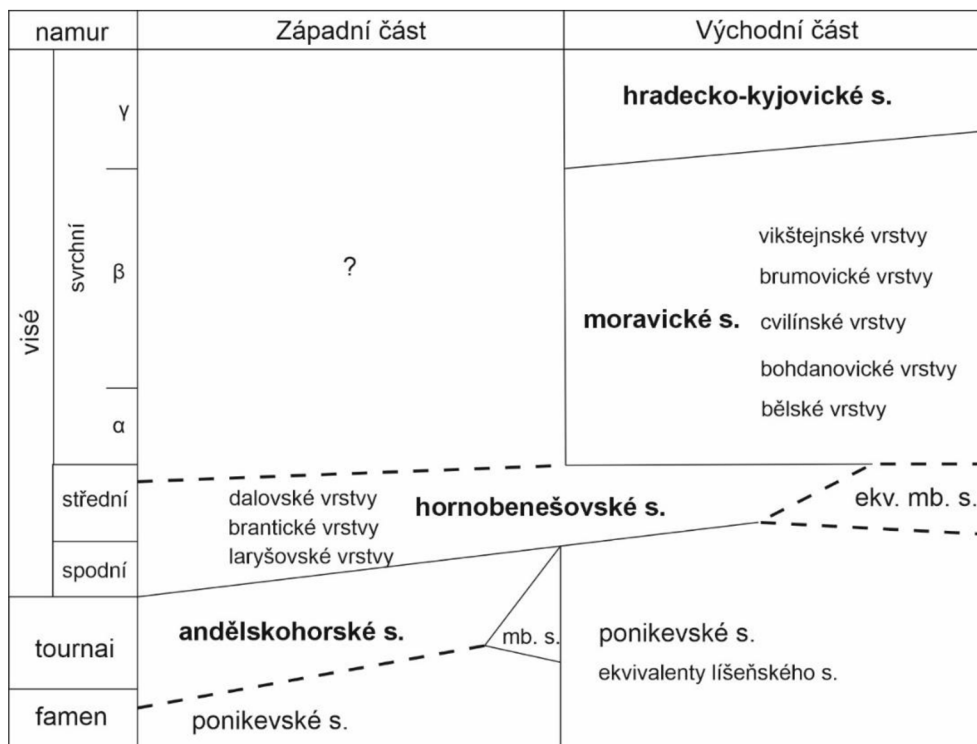
Obr. 4: Stratigrafický přehled nizkojesenického kulmu (Zapletal et al., 1989). (mb.s. - moravskoberounské souvrství).
