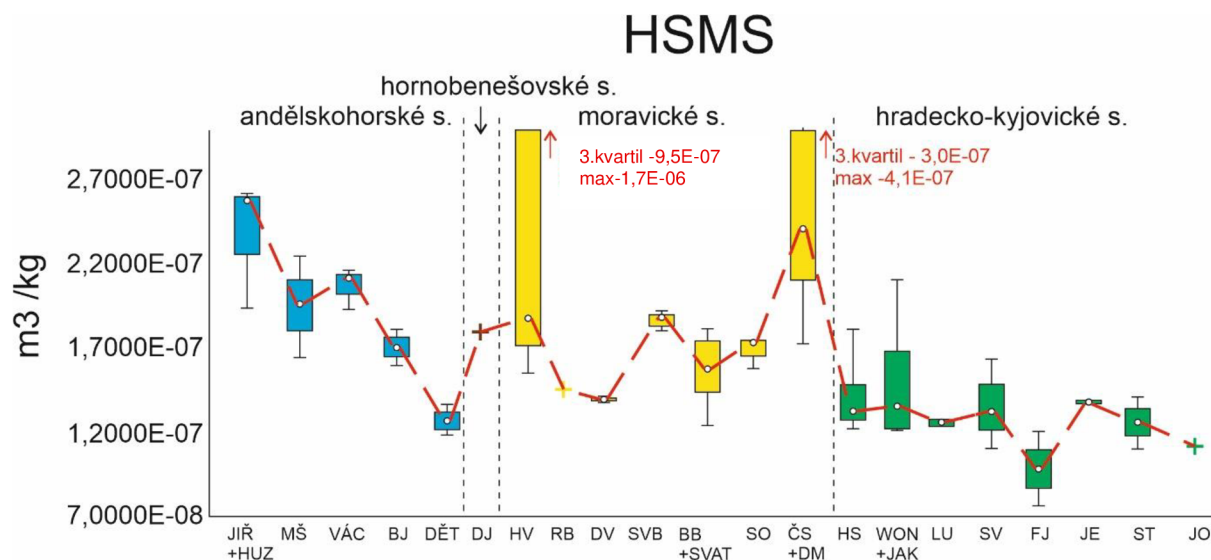
Obr. 6: Výsledky hmotnostně specifické magnetické susceptibility. Zkoumané lokality jsou seřazeny podle stratigrafie od nejstarších (andělskohorské souvrství) po nejmladší (hradecko-kyjovické souvrství). Zkratky lokalit odpovídají Tab. 1.
