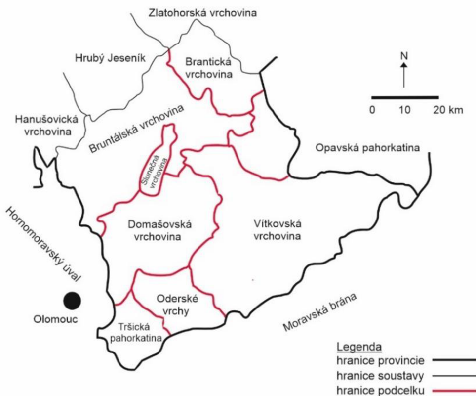
Obr. 2: Geomorfologické podcelky Nízkého Jeseníku podle Demka a Mackovčina (2006).
