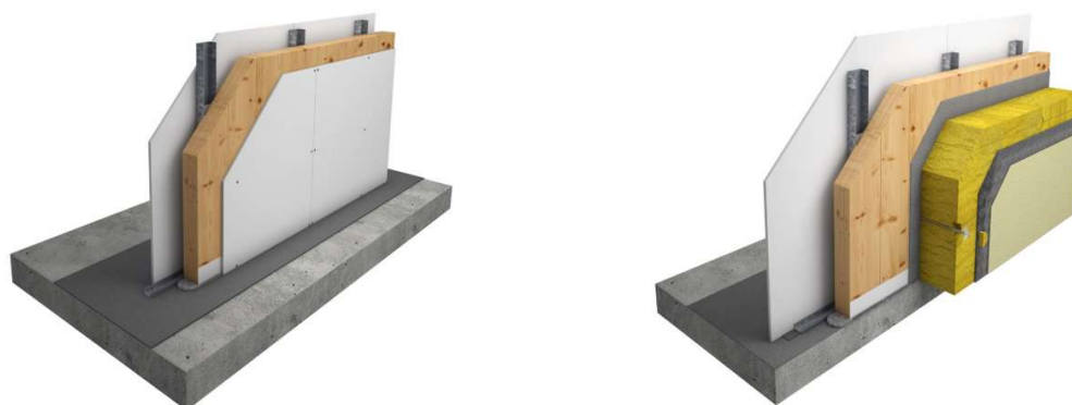
Obrázek 21 - Stěnové panely DEKPANEL (Zdroj: [30])
