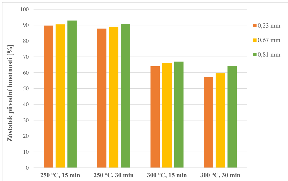
Obrázek 19: Vliv velikosti částic pilin z borovice na změnu hmotnosti při torefakci [55, 64].
