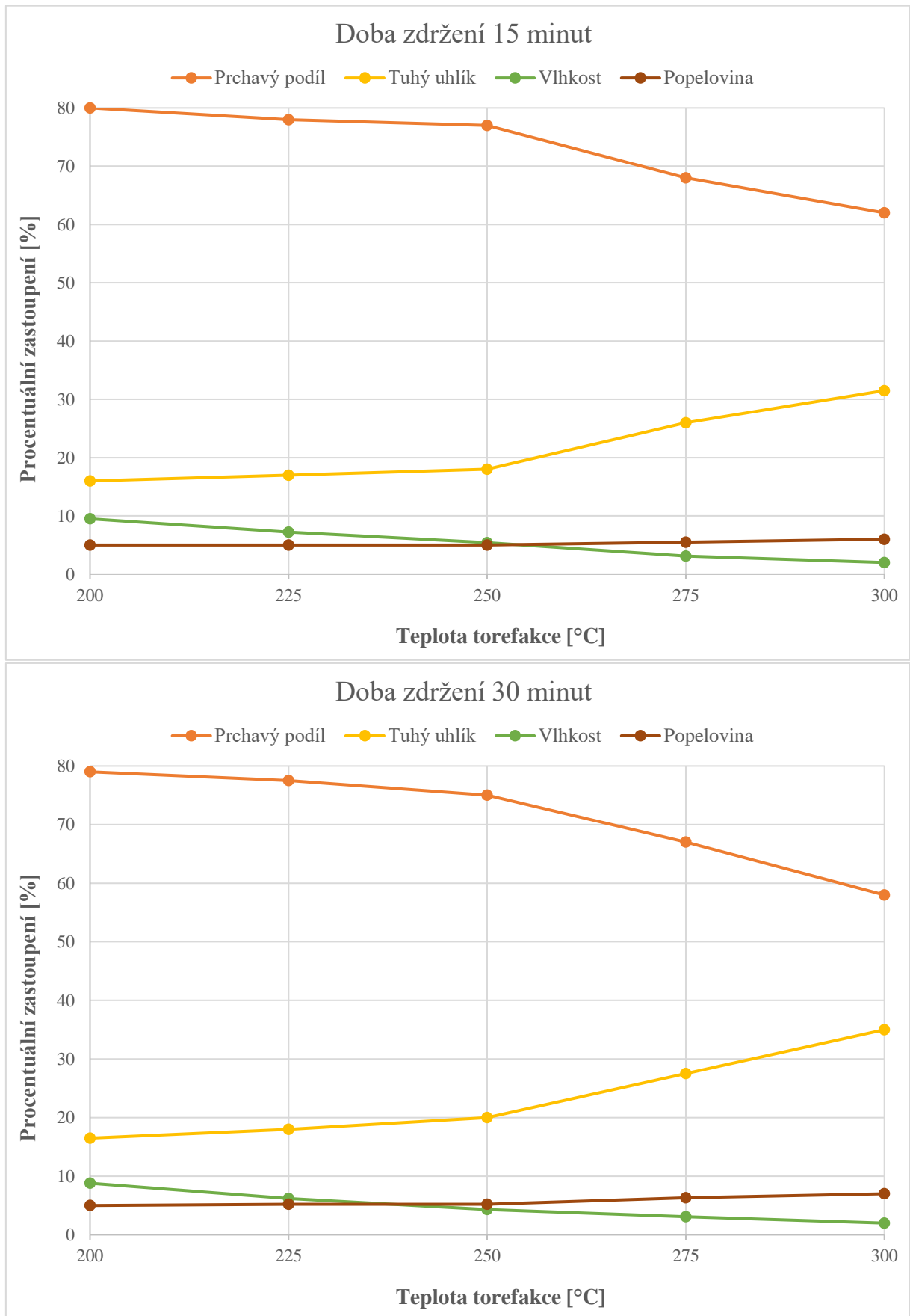
Obrázek 16: Vliv teploty a doby zdržení na hrubý rozbor bagasy z cukrové třtiny (1/2) [62].
