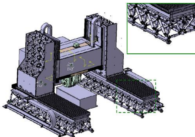
Obr. 9 Prototyp nosné části od firmy Fatronik [66]
