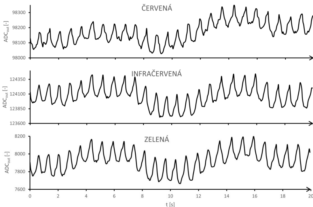
Obrázek 3.9 Průběhy dat ze senzoru při měření na čele.
