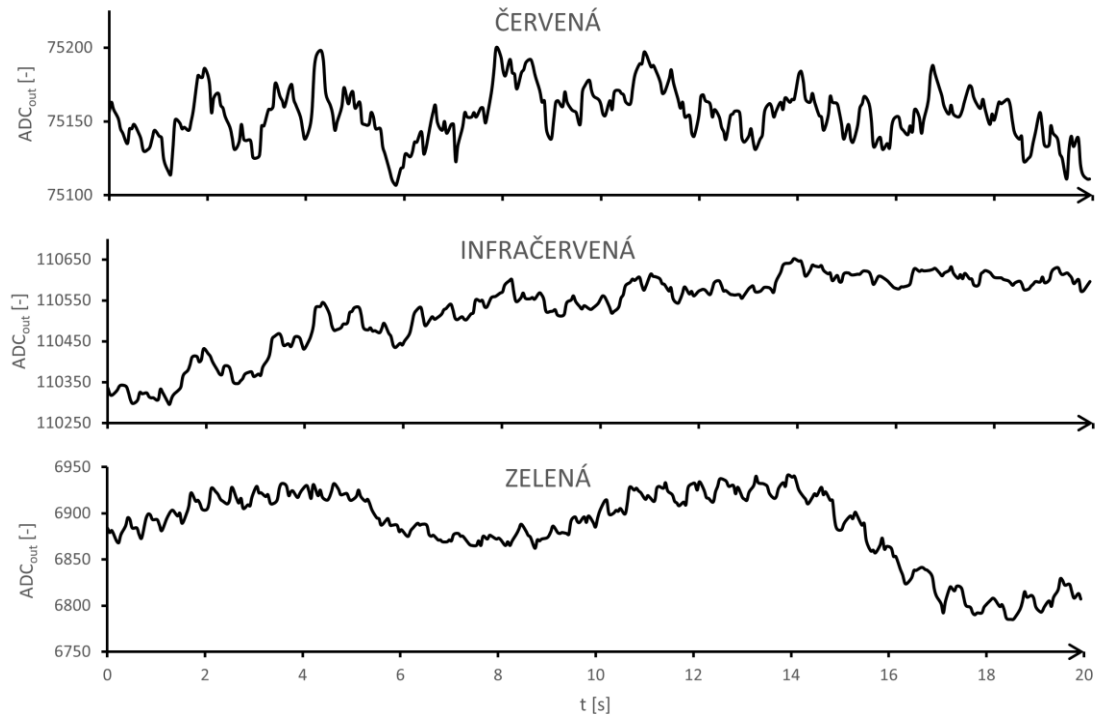
Obrázek 3.8 Průběhy dat ze senzoru při měření nad kotníkem.
