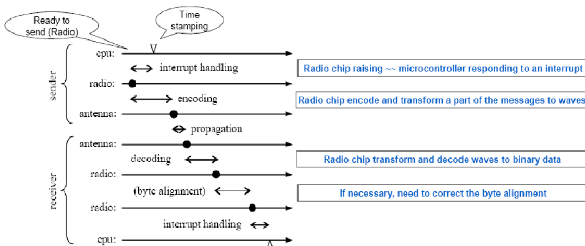
Obrázek 1.5: Zdroje chyb časové synchronizace. [24]
