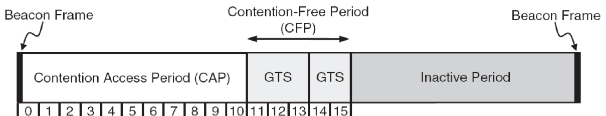
Obrázek 2.10 Superrámec [7]
