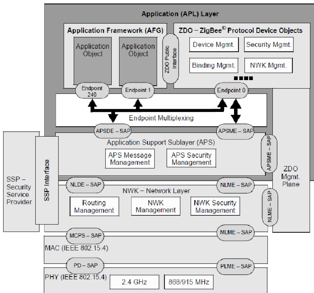
Obrázek 2.2: Architektura ZigBee [5]
