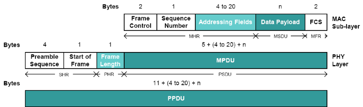
Obrázek 2.9 Datový rámec [8]
