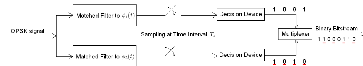
Obrázek 2.8 Schéma demodulace O-PSK [9]
