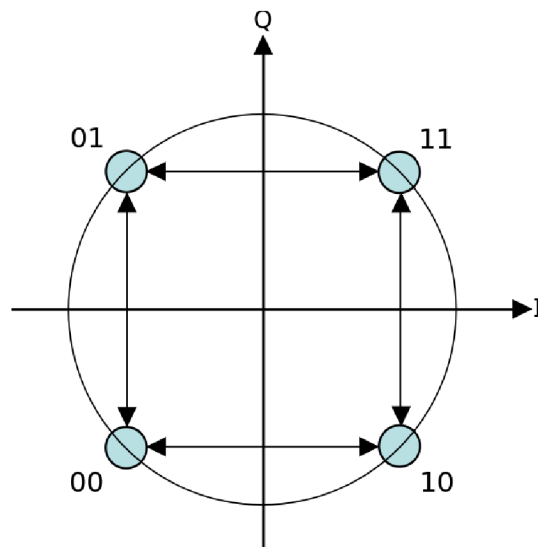
Obrázek 2.6 Konstelační diagram modulace O-PSK. [9]
