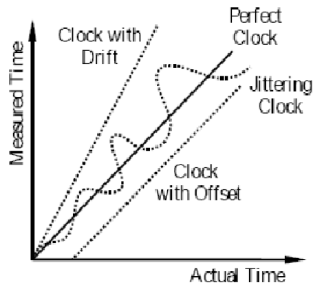
Obrázek 1.3: Měření času a chyby hodin. [23]
