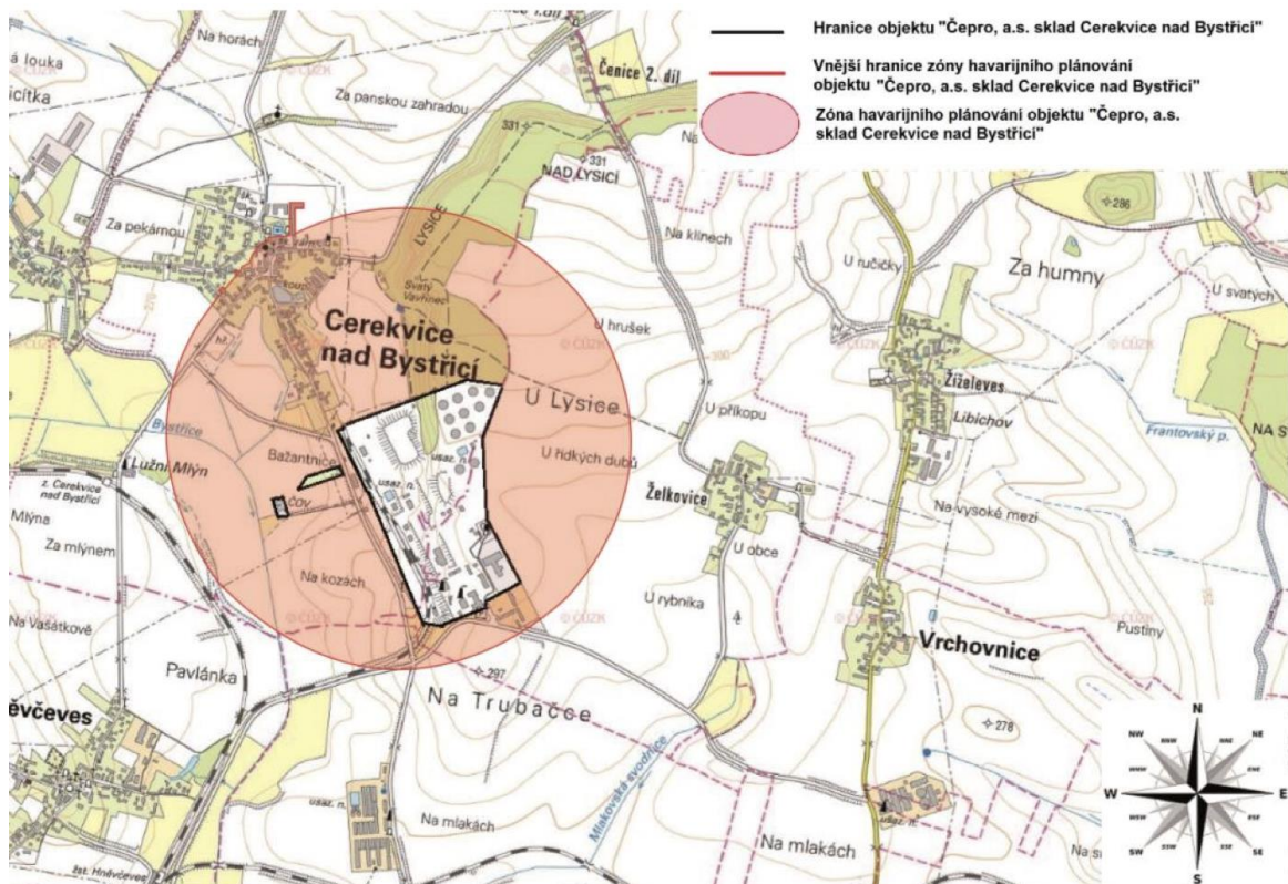
Obrázek 2 Zóna havarijního plánování, pro kterou je zpracován havarijní plán
