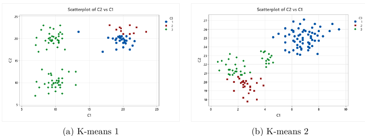
Obrázek 2.28: K-means - Minitab
