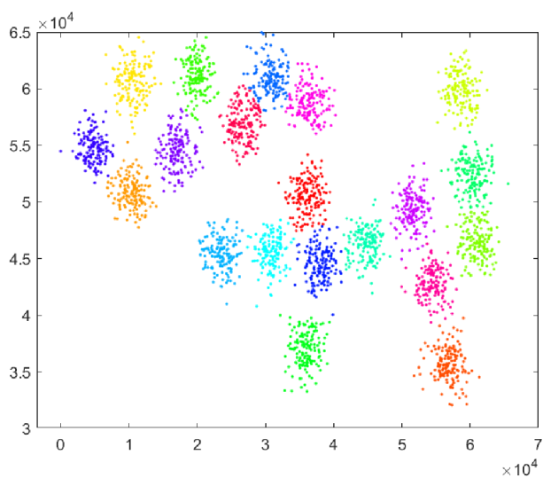
Obrázek 2.13: K-means 8 - MATLAB
