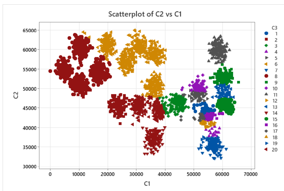
Obrázek 2.28: K-means - Minitab
