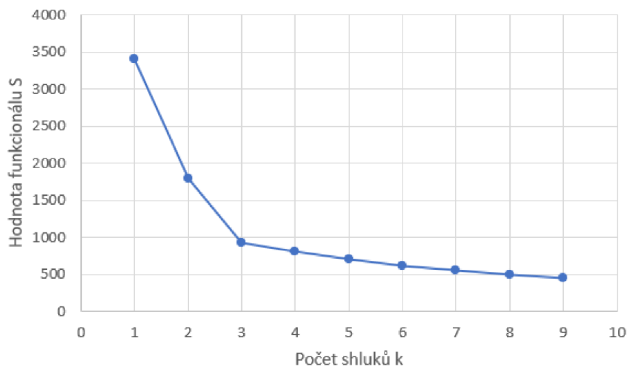
Obrázek 1.4: Elbow method
