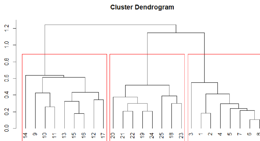
Obrázek 2.15: Dendrogram 3 - R
