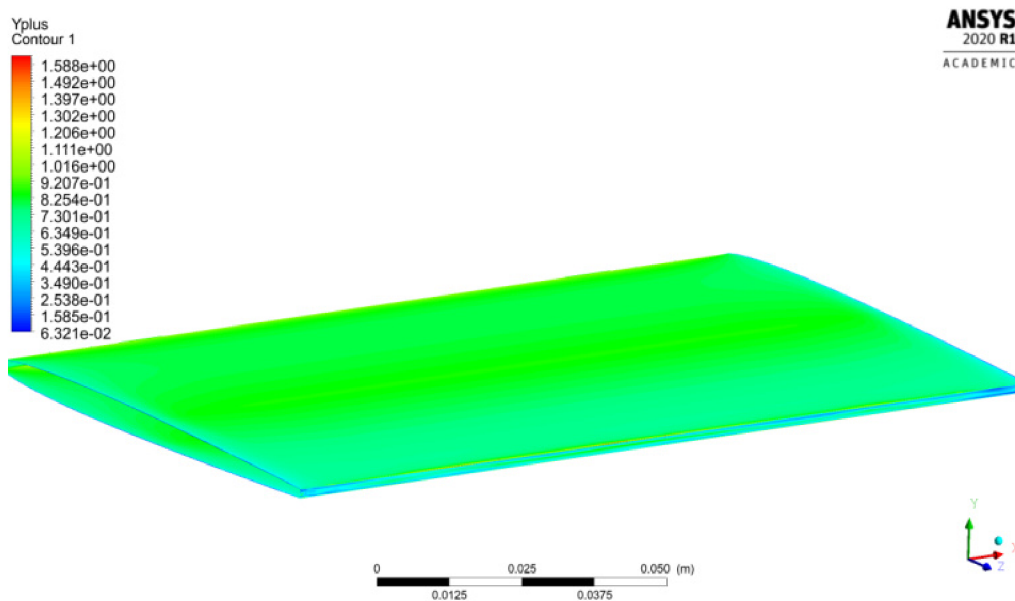
Obr. 5.15: Hodnota veličiny y^+ na stěnách lopatky, ukážka pro 15 m/s.
