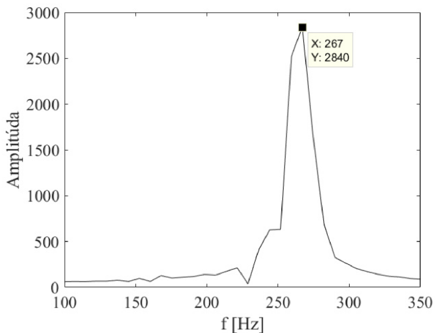
Obr. 5.36: FFT, vibrácie/koefficient vztlaku, simulácia 2,5 m/s uhol nábehu 0^\circ .
