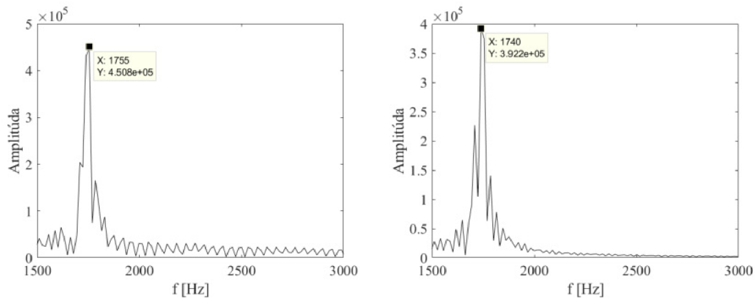
Obr. 5.17: FFT z počítaných hodnôt pulzácií tlaku (vľavo) a koeficientu vztlaku (vpravo), ukážka pre 15 m/s uhol nábehu 0°.
