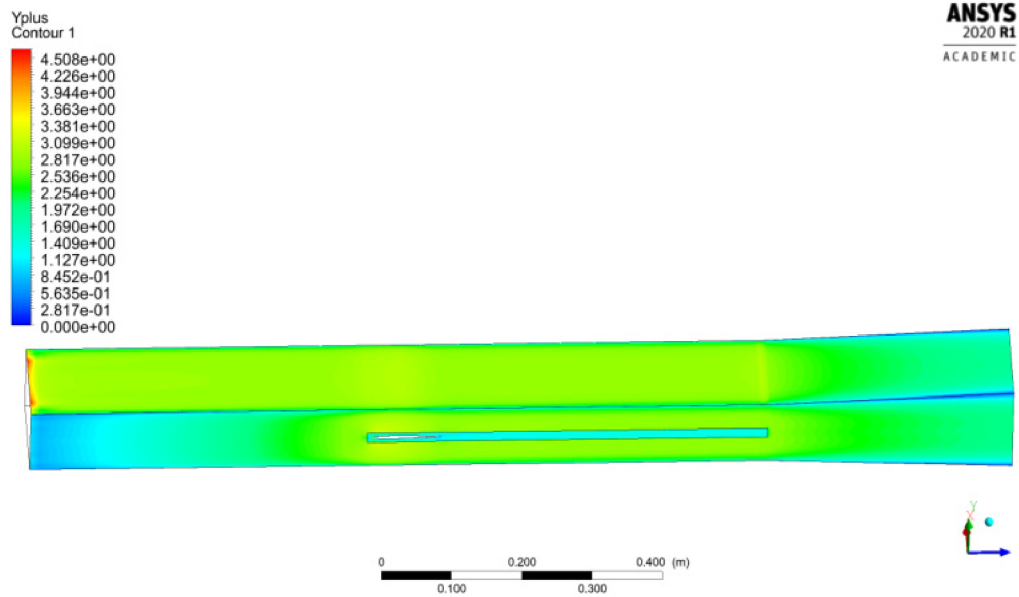
Obr. 5.14: Hodnota veličiny y^+ na stěnách domény, ukážka pro 15 m/s.
