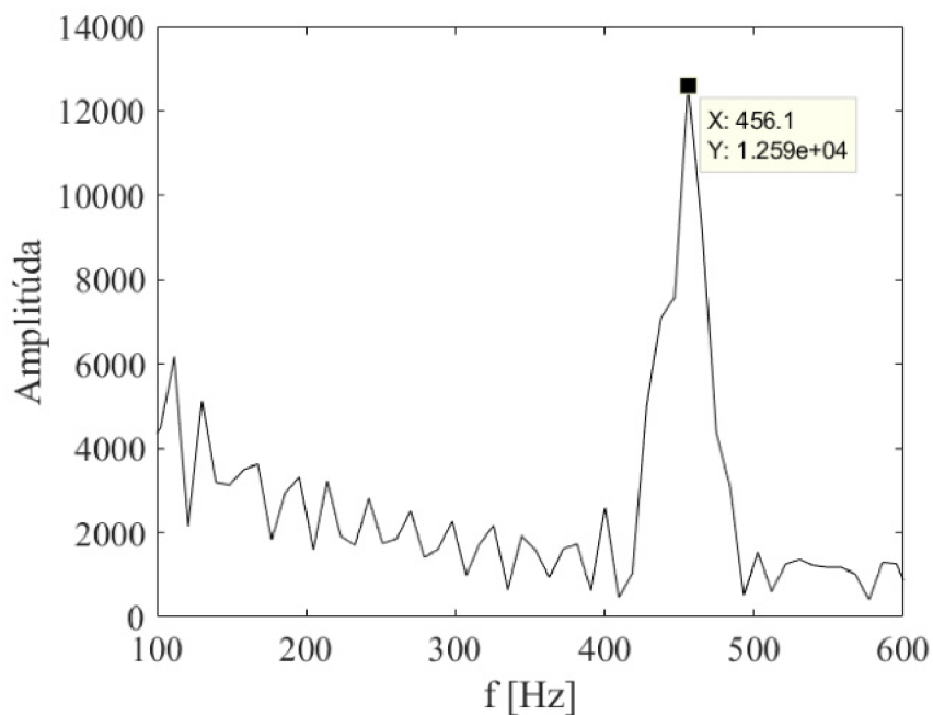
Obr. 5.52: FFT, vibrácie/koefficient vztlaku, simulácia 5 m/s uhol nábehu 5^\circ .
