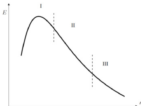
Obr. 1.4: Spektrum turbuletnej kinetickej energie. Prevzaté a upravené z [6].
