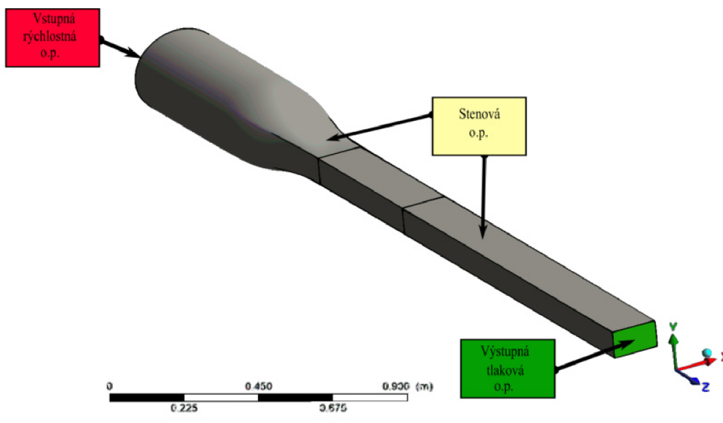
Obr. 4.5: Priradenie okrajových podmienok pre doménu.
