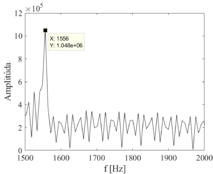
Obr. 5.19: FFT pulzácie tlaku pre simuláciu SST k - \omega , 15 m/s uhol nábehu 0^\circ .
