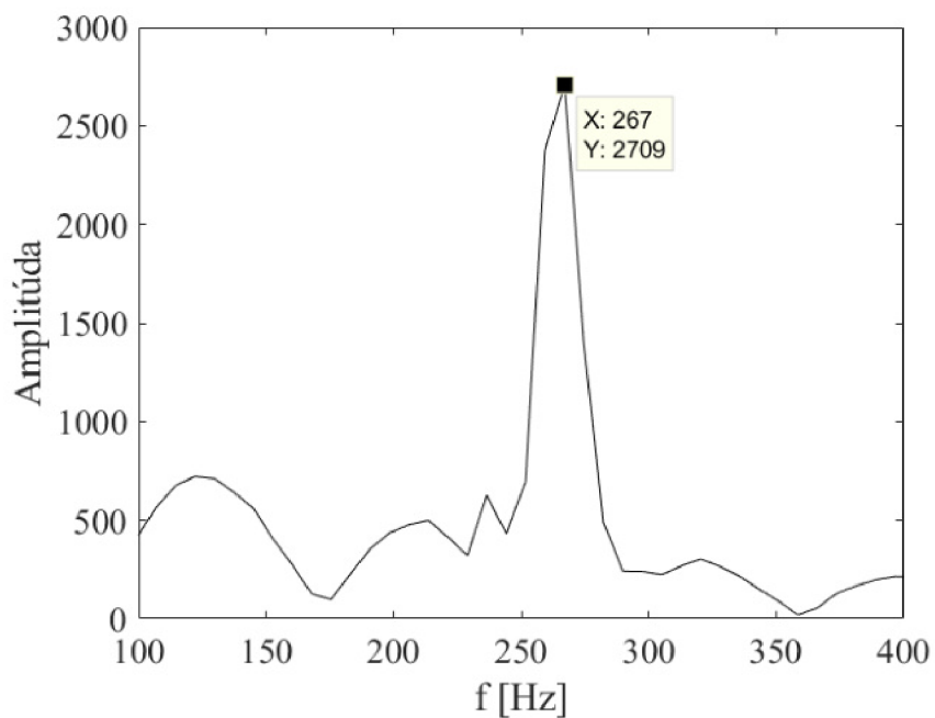
Obr. 5.37: FFT, tlakové pulzácie, simulácia 2,5 m/s uhol nábehu 0^\circ .
