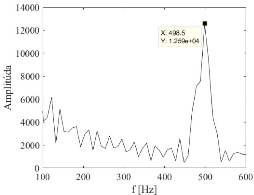
Obr. 5.53: FFT, tlakové pulzácie, simulácia 5 m/s uhol nábehu 5^\circ .
