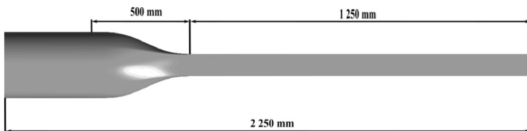
Obr. 4.2: Geometria priváděcí části.
