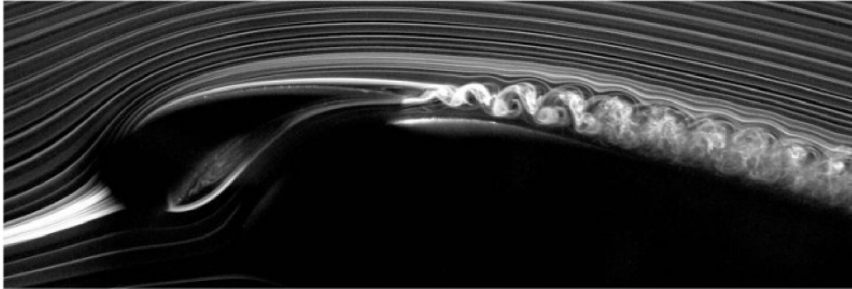
Obr. 1.10: Kármánová vírová cesta pri obtekaní lopatky. Prevzaté z [20].
