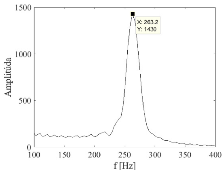
Obr. 5.21: FFT pulzácie tlaku pre simuláciu SST k - \omega , 2,5 m/s uhol nábehu 0^\circ .
