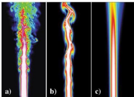
Obr. 2.3: Porovnanie simulácie DNS (a) LES (b) a RANS (c). Prevzaté a upravené z [22].
