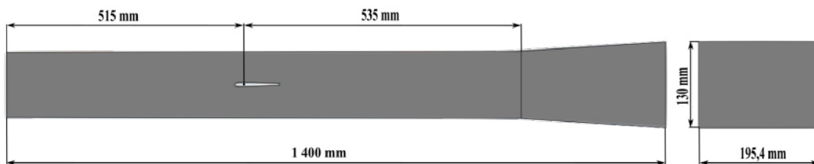
Obr. 5.2: Geometria výpočtovej domény.
