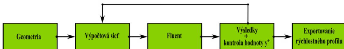
Obr. 4.1: Schéma postupu výpočtu pro priváděcí část.
