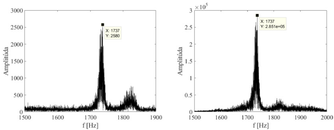
Obr. 5.18: FFT z meraných hodnôt pulzácií tlaku (vľavo) a vibrácií (vpravo), ukážka pre 15 m/s uhol nábehu 0°.
