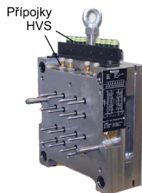
Obr. 8.2 Elektrické připojky na horké polovině formy [20]
