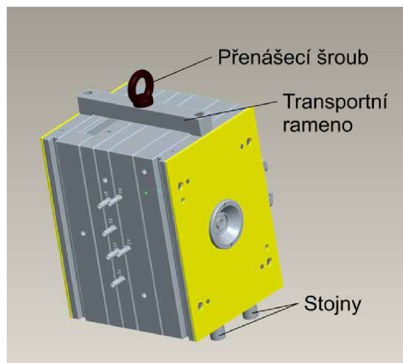
Obr. 8.33 Vstřikovací forma - přenašecí prvky
