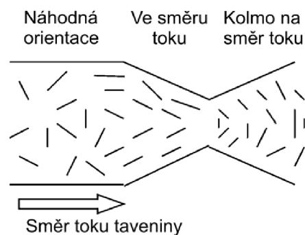
Obr. 6.2 Natočení vláken nebo molekul podle změny průřezu [29]
