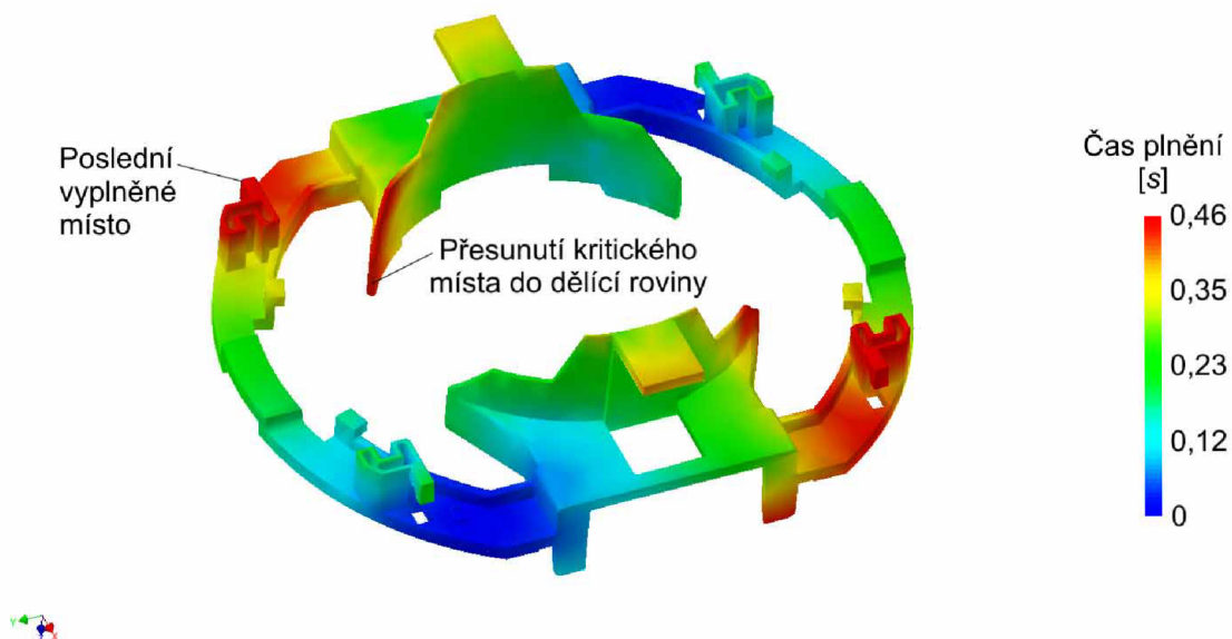
Obr. 8.20 Čas plnění - po posunutí vtoků
