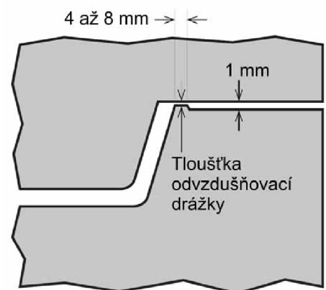
Obr. 4.16 Odvzdušňovací drážka [40]
