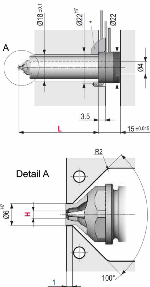
Obr. 8.11 Schéma zvoleného typu externě vytápěné horké trysky [57]
