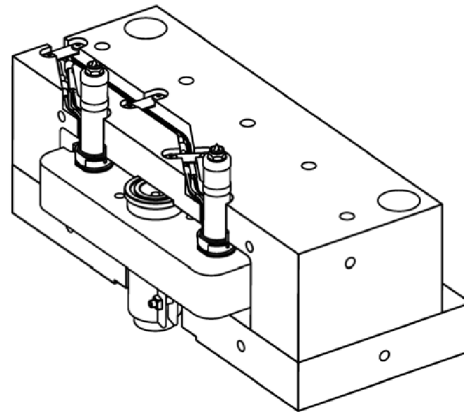
Obr. 7.7 Externě vyhřívaná horká vtoková soustava, řez horkou polovinou formy [42]
