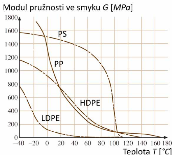
Obr. 3.16 Modulus pružnosti vs. teplota [25]
