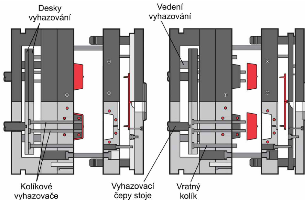
Obr. 4.15 Třidedková vícenásobná forma, pohyb a popis vyhazovacího systému [40]
