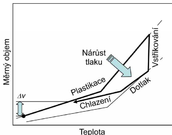
Obr. 4.8 Zhušťování polymeru během Formování [1]
