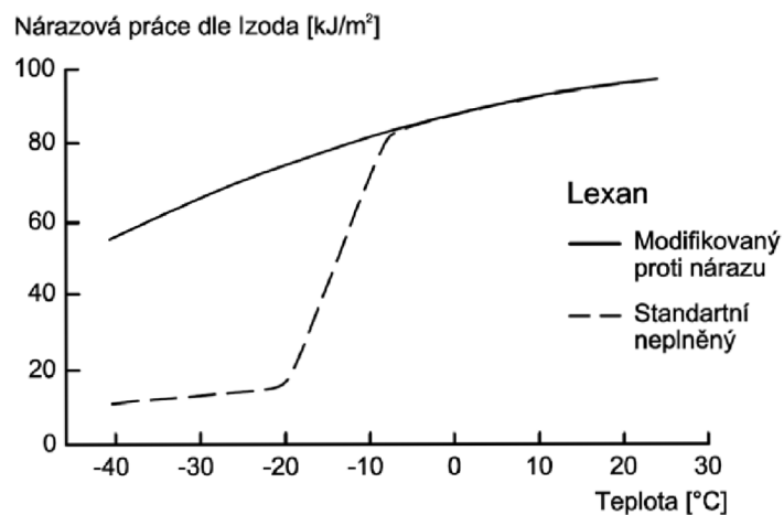
Obr. 3 Nárazová práce Lexanu vs. teplota [51]
