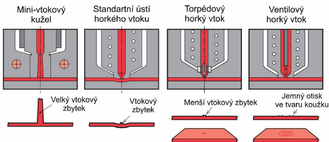
Obr. 5.6 Typy vtokových ústí externě vyhříváných horkých trysek [40]
