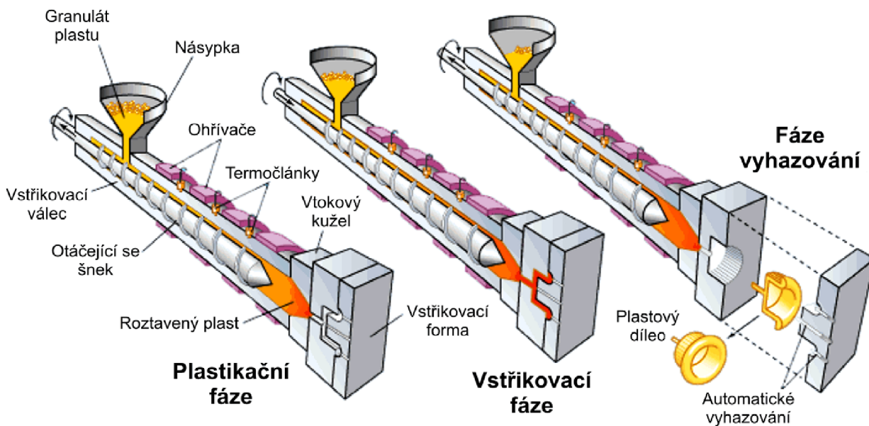
Obr. 4.4 Vstřikovací cyklus [62]
