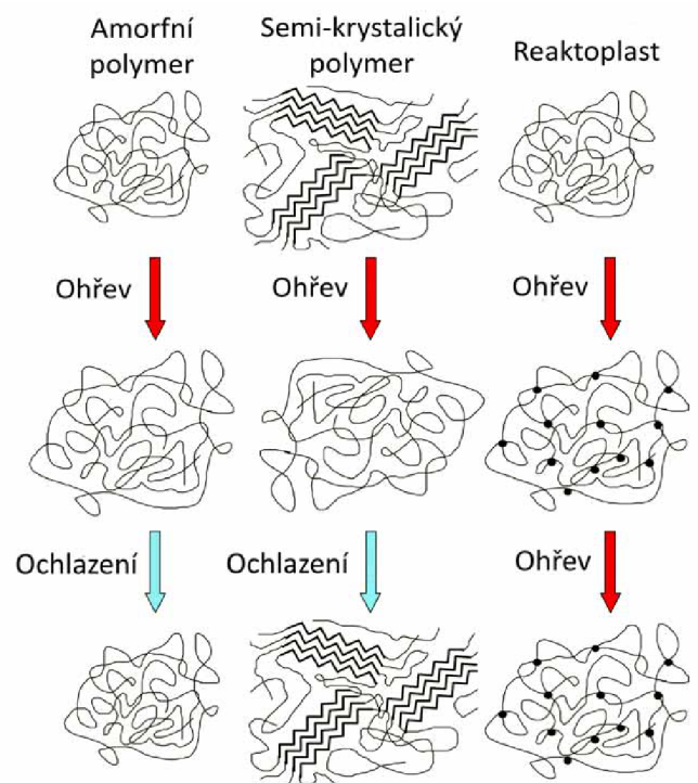
Obr. 3.6 Mikrostruktura plastů [38]
