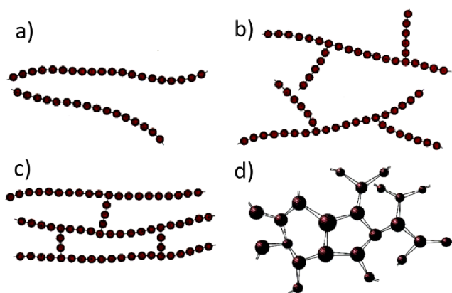
Obr. 3.3 Molekuly plastů [21]
