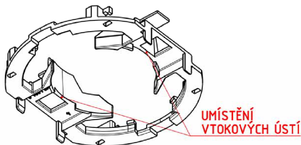
Obr. 7.2 Umístění vtokových ústí vzhledem ke tvaru plastového dílce
