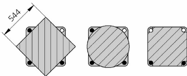
Obr. 9.3 Použitelná plocha stolu po vyjmutí sloupů [4]
