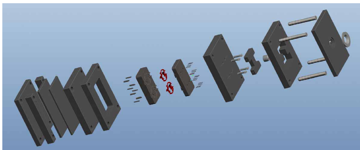
Obr. 8.12 Návrh vstříkovací formy, rozložený 3D pohled
