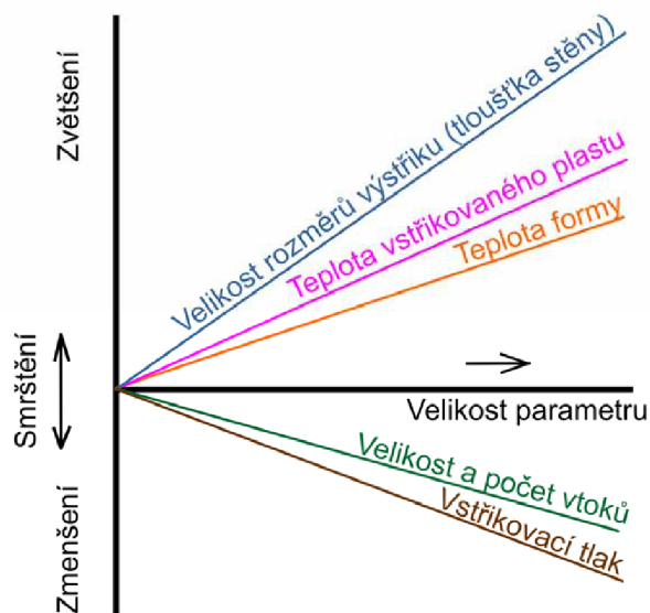
Obr. 3.12 Vliv vybraných činitelů na velikost smrštění [11]
