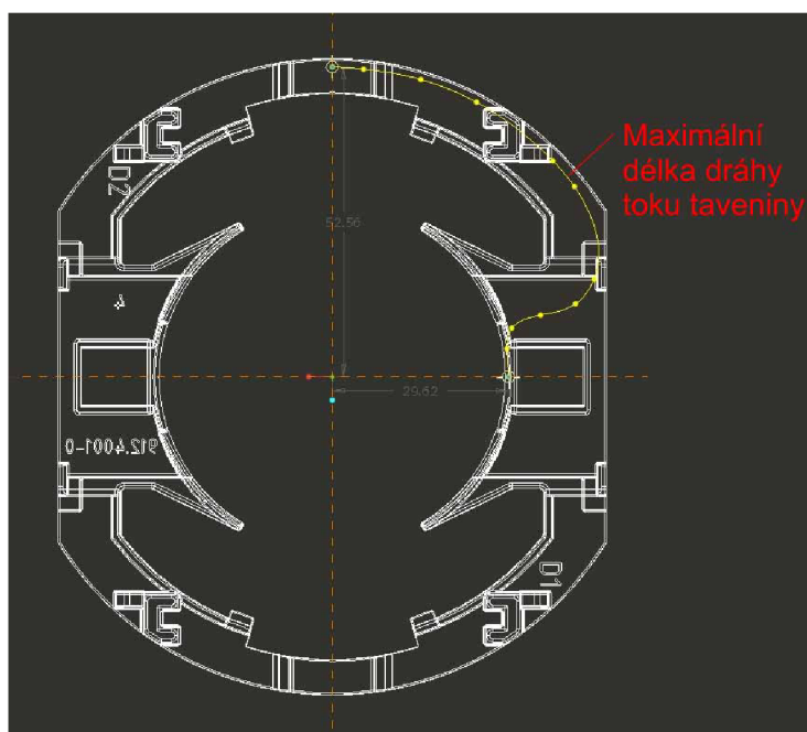
Obr. 8.14 Maximální dráha toku taveniny vyznačená žlutou křivkou
