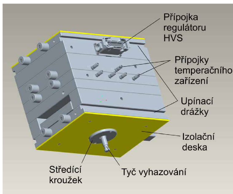
Obr. 8.34 Vstřikovací forma - upínací a připojovací prvky
