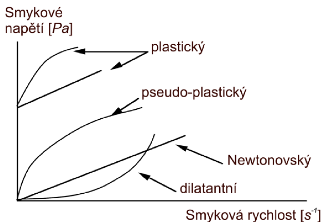
Obr. 7.6 Tokové modely různých druhů tekutin [60]
