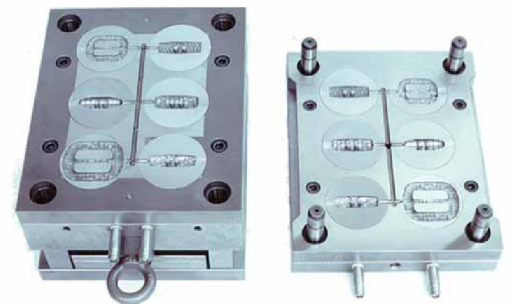
Obr. 4.19 Vstřikovací forma [39]
