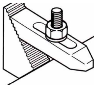
Obr. 9.4 Stupňovitá upínka [44]
