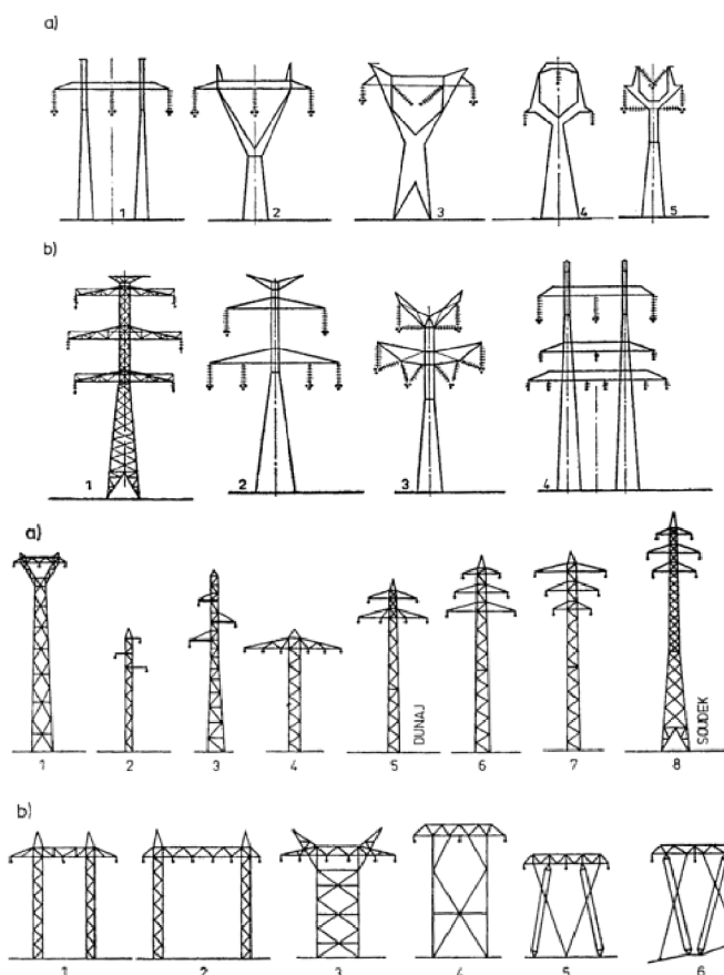
Obr. 1.2 Typy stožáru [3]
