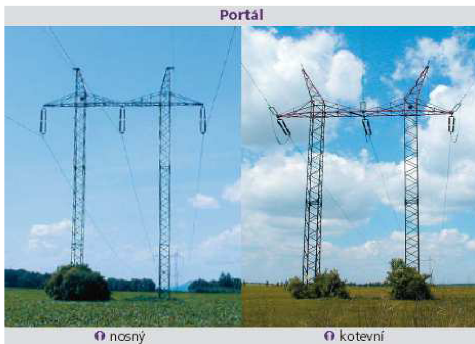
Obr. 1.6 Portálový stožár [1]
