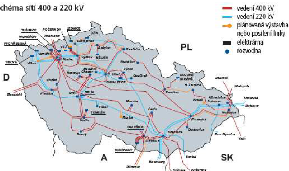
Obr. 1.1 Přenosová soustava [1]
