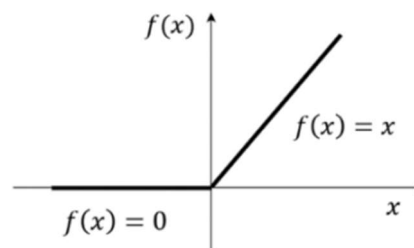
Fig. 8 - ReLU function
