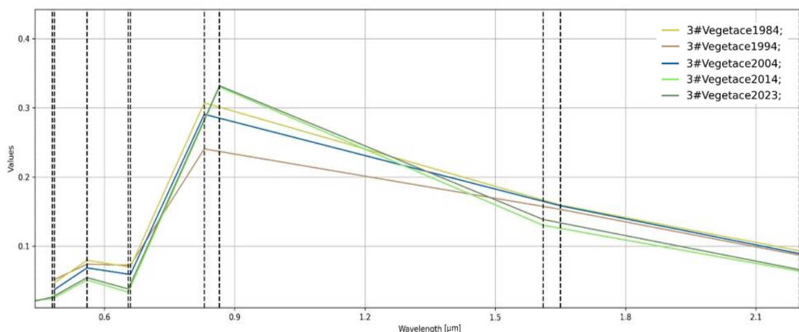
Obr. 14: Spektrální křivka odrazivosti vegetace v okolí skládky TKO Zábřeh
