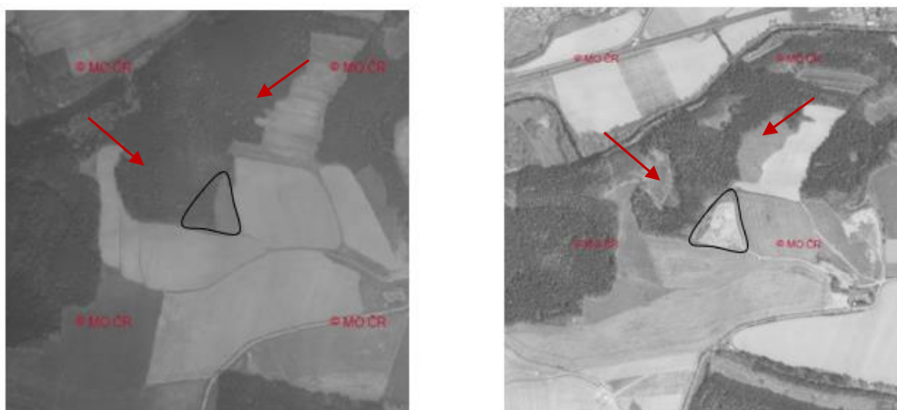
Obr. 9: Ortofotomapy ukazující na změnu lesního porostu severozápadně od skládky TKO Zábřeh (vlevo 1968, vpravo 1993). Zdroj: ags.cuzk.cz
