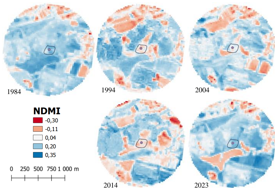
Obr. 11: NDMI pro skládku Zábřeh (shora zleva – 1984, 1994, 2004, 2014, 2023)
