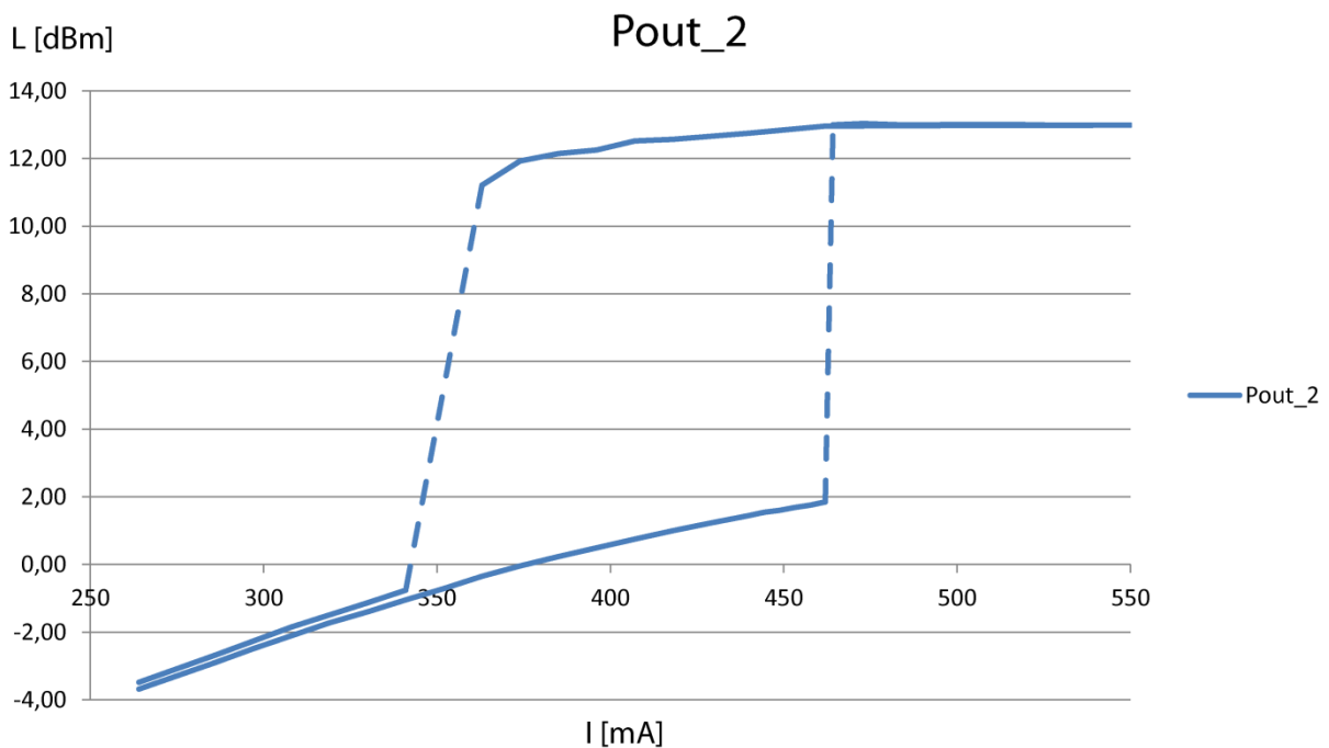
Obr. 18 Výkonová hysterézná krivka SOA zosilňovača. Meranie z výstupu generátoru s kalibrovaným útlmovým článkom 5 dBm, vstupný výkon= -2,35 dBm. Smernica nábežnej časti krivky: 0,0271.
