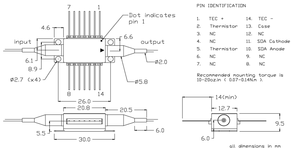
Obr. 15 Rozmery a usporiadanie pinov u SOA1013
