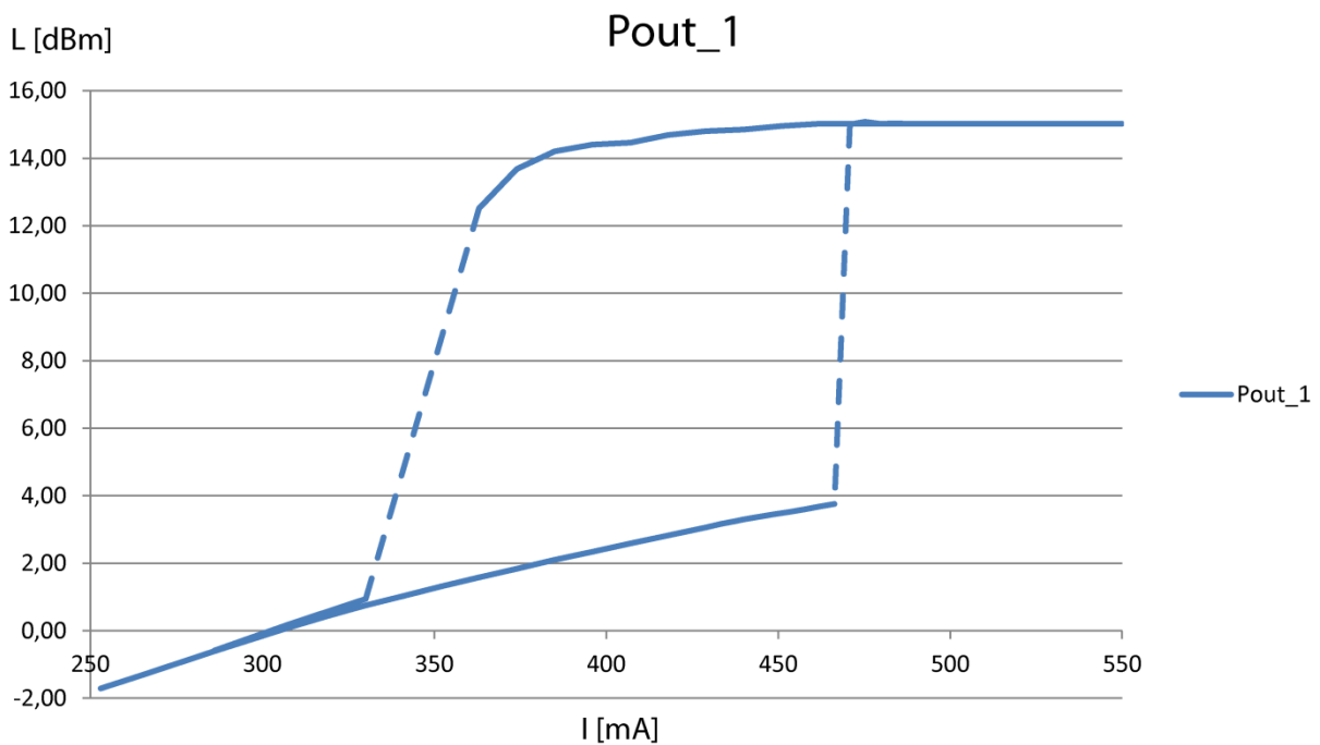
Obr. 17 Výkonová hysterézná krivka SOA zosilňovača. Meranie z výstupu generátoru bez útlmového článku, vstupný výkon= 2,24 dBm. Smernica nábežnej časti krivky: 0,0248.
