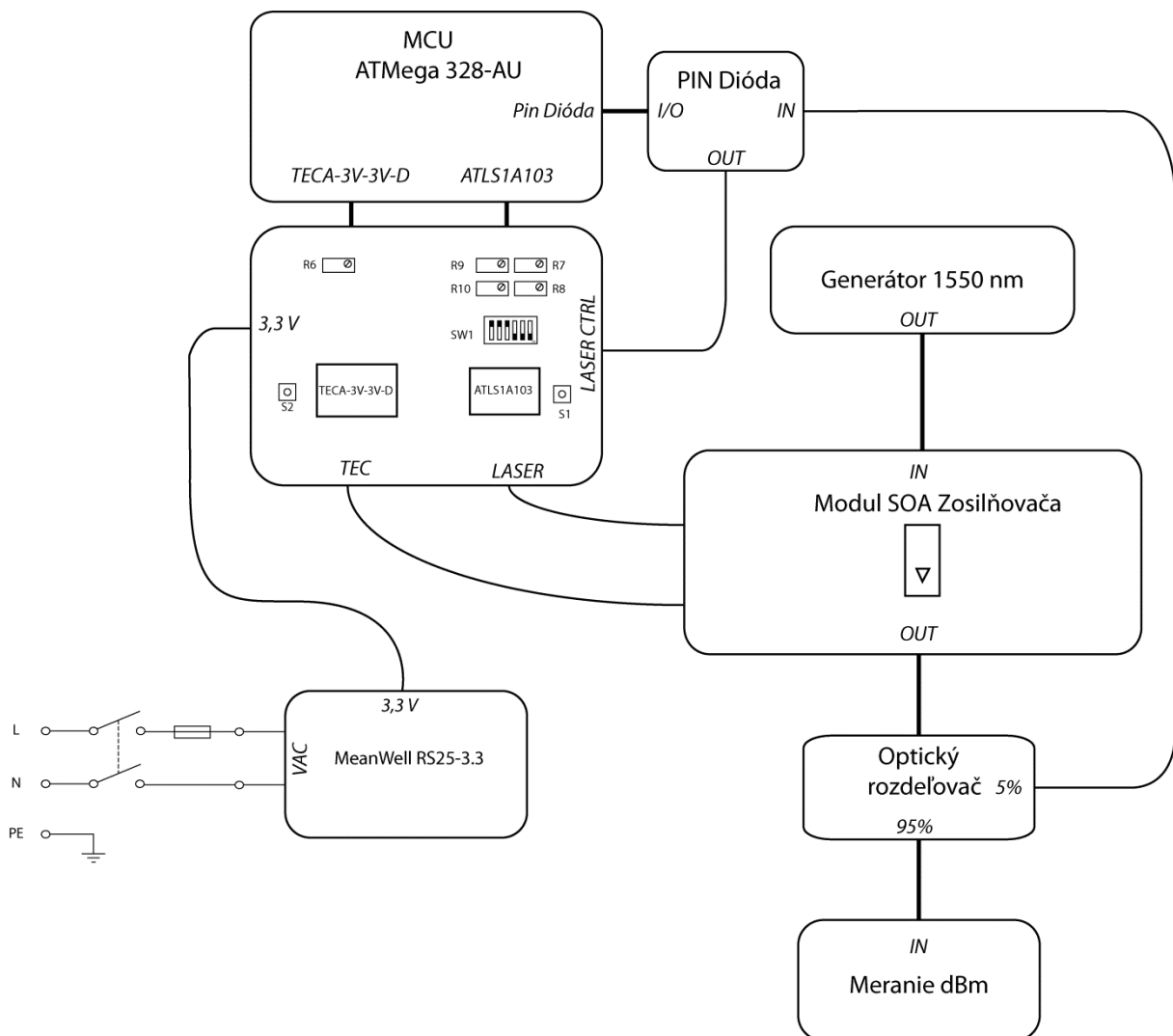
Obr. 11 Zapojenie modulu optického zosilňovača SOA s digitálnym riadením
