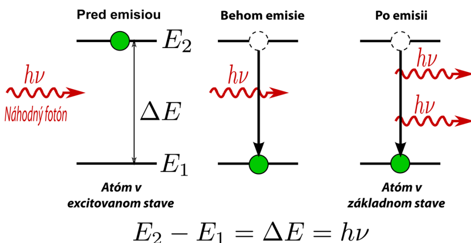
Obr. 7 Absorpcia, spontánna emisia a stimulovaná emisia v SOA zosilňovači
