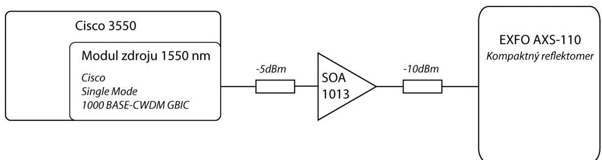
Obr. 16 Ukážka zapojenia merania pomocou kompaktného reflektomeru EXFOAXS-110 použitého pri meraní hysteréznej slučky SOA.
