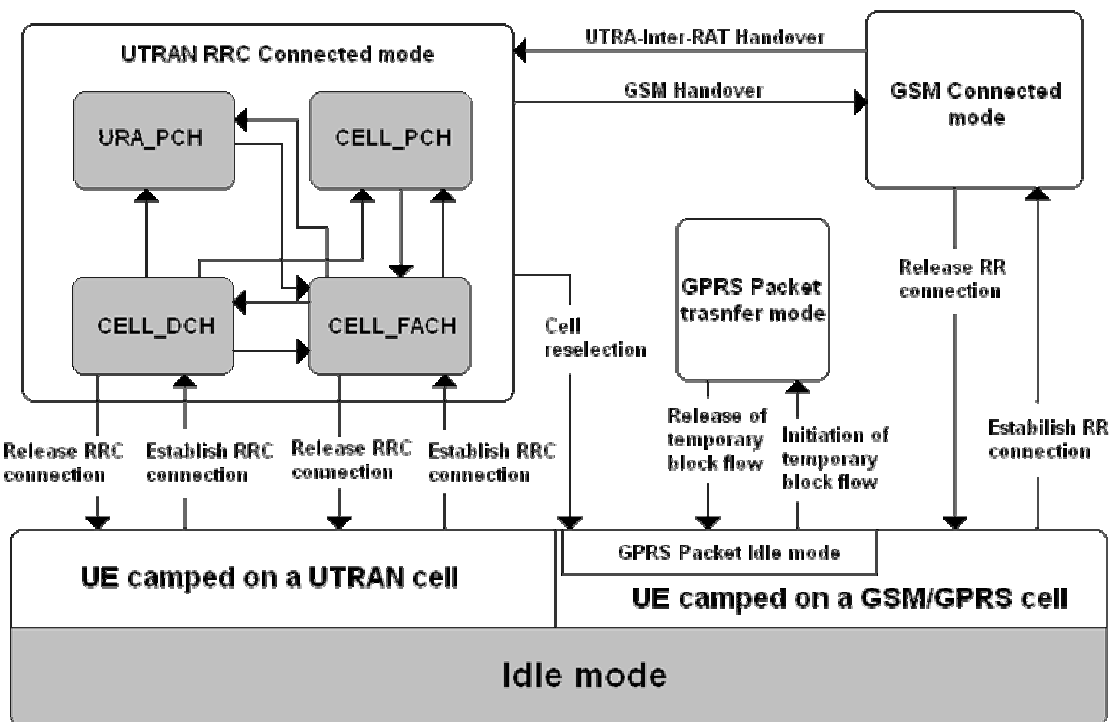
Obr. 9.3: Stavby RRC a přechody mezi nimi
