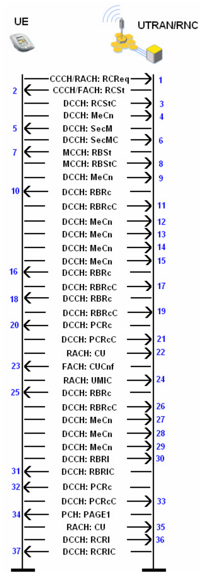
Obr. 4.7: Průběh komunikace mezi UE a UTRAN/RNC při datové službě
