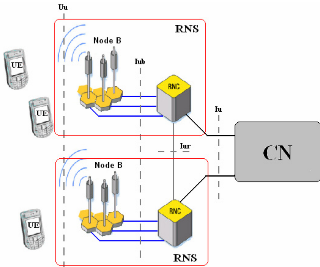
Obr. 2.7: Architektura UTRAN
