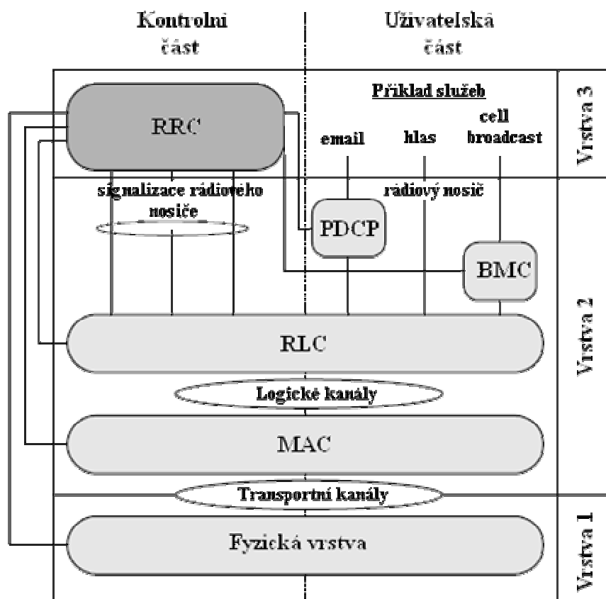
Obr. 9.1: Protokolová architektura
