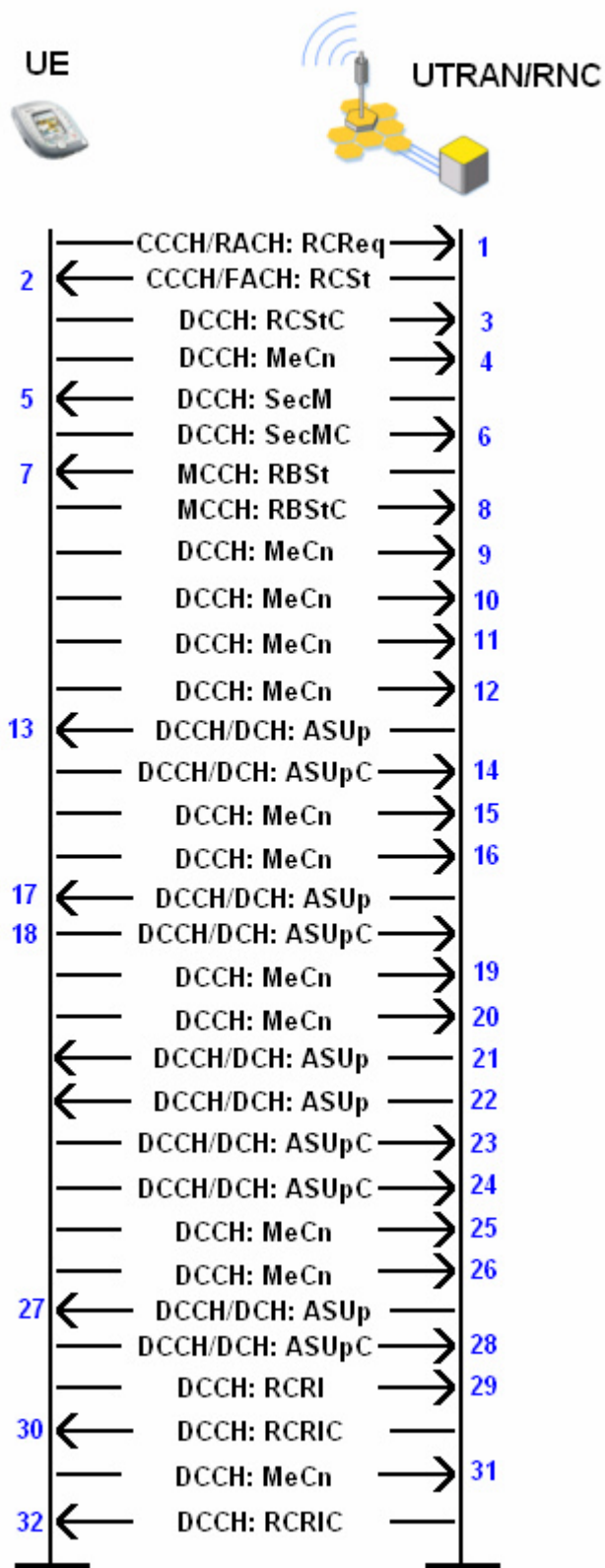
Obr. 4.6: Průběh komunikace mezi UE a UTRAN/RNC při hovorové službě
