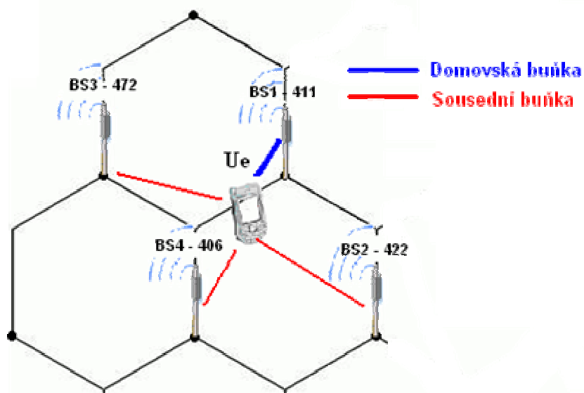
Obr. 8.7: FDD buňky v Idle stavu a jejich výběr
