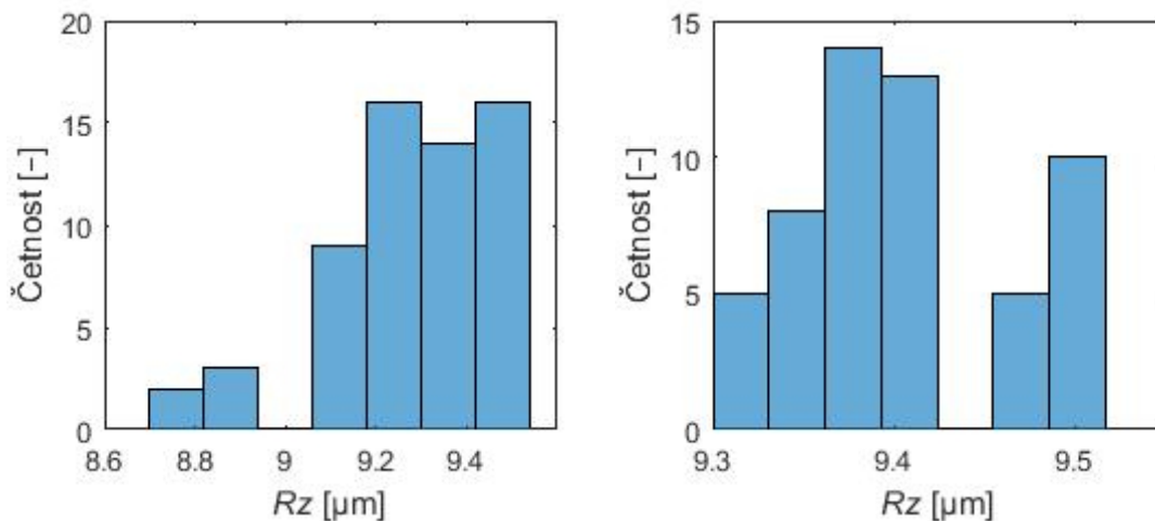
Obr. P15) Histogramy souborů hodnot parametru Rz , měření A2_R12,5 (vlevo) a A2_R40 (vpravo)
