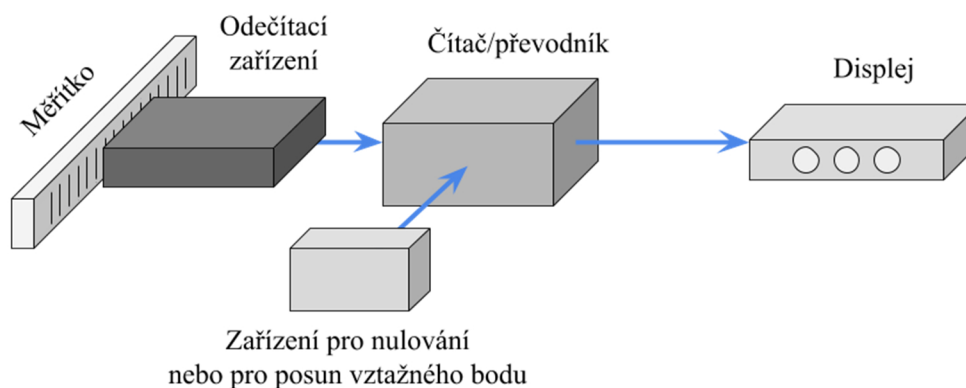
Obr. 23) Obecné schéma odměřovacího systému (upraveno z [21])
