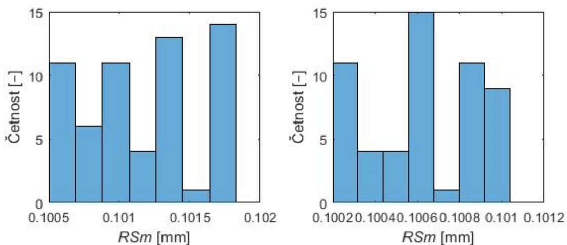
Obr. P17) Histogramy souborů hodnot parametru RSm , měření A2_R12,5 (vlevo) a A2_R40 (vpravo)
