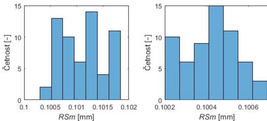
Obr. P16) Histogramy souborů hodnot parametru RSm , měření A1_R12,5 (vlevo) a A1_R40 (vpravo)
