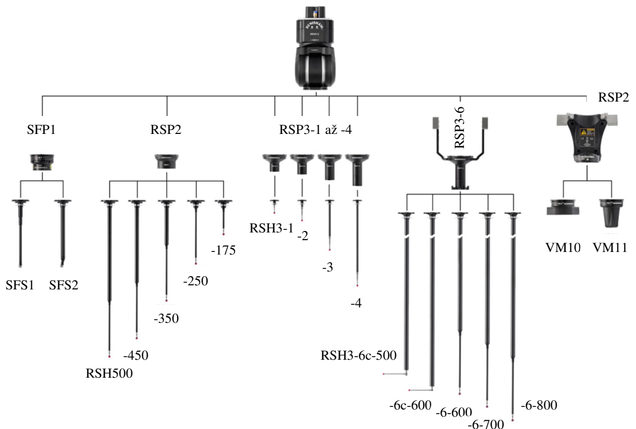
Obr. 25) Hlavice, sondy a nástavce systému REVO (na obrázku starší sonda měření textury povrchu SFP1, upraveno z [31])
