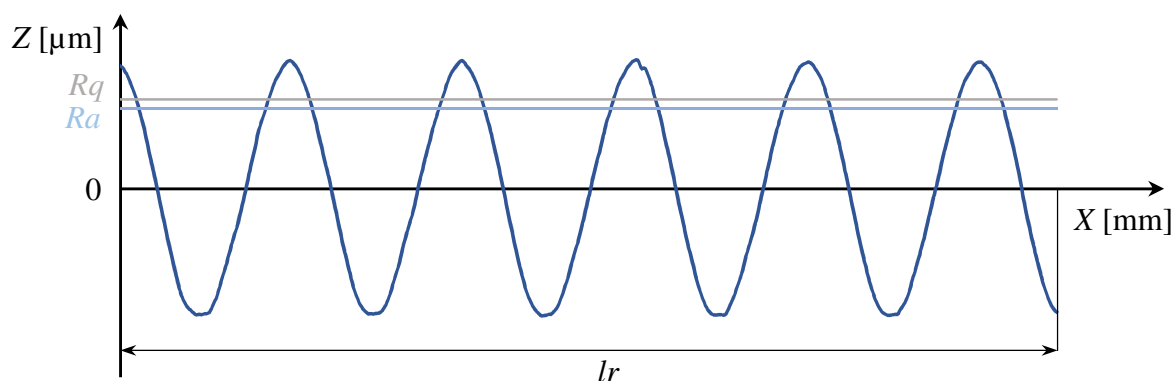
Obr. 8) Průměrná aritmetická úchylka profilu drsnosti Ra a průměrná kvadratická úchylka profilu drsnosti Rq na periodickém povrchu
