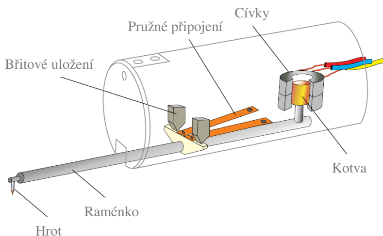
Obr. 17) Schéma indukčnostního měřicího systému (snímače; upraveno z [2])
