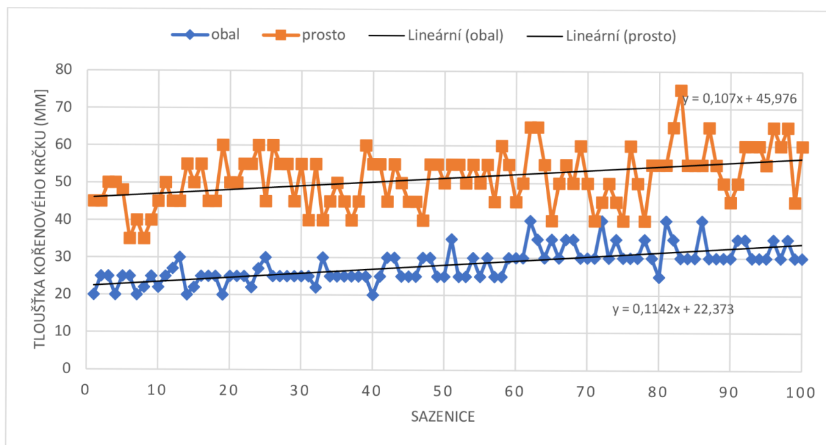
Graf 14 Tloušťka kořenového krčku pětiletých sazenic (obalovaná, prostokořenná)
