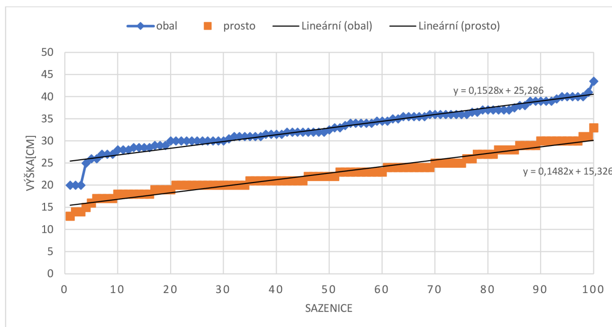
Graf 3 Přírůst jednoletých sazenic (obalovaná, prostokořenná) Zdroj: vlastní zpracování
