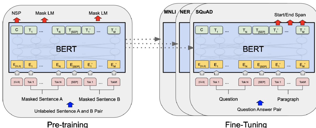
Obrázek 3.4: BERT, převzato z [14].
