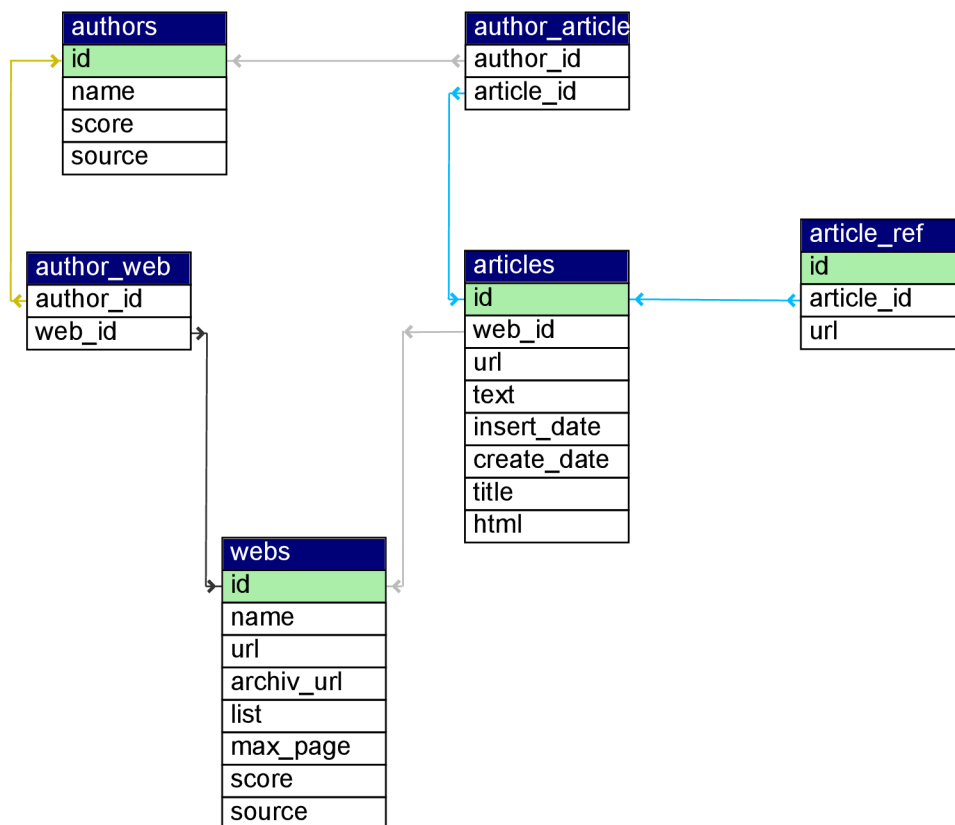
Obrázek 5.3: Schéma databáze.
